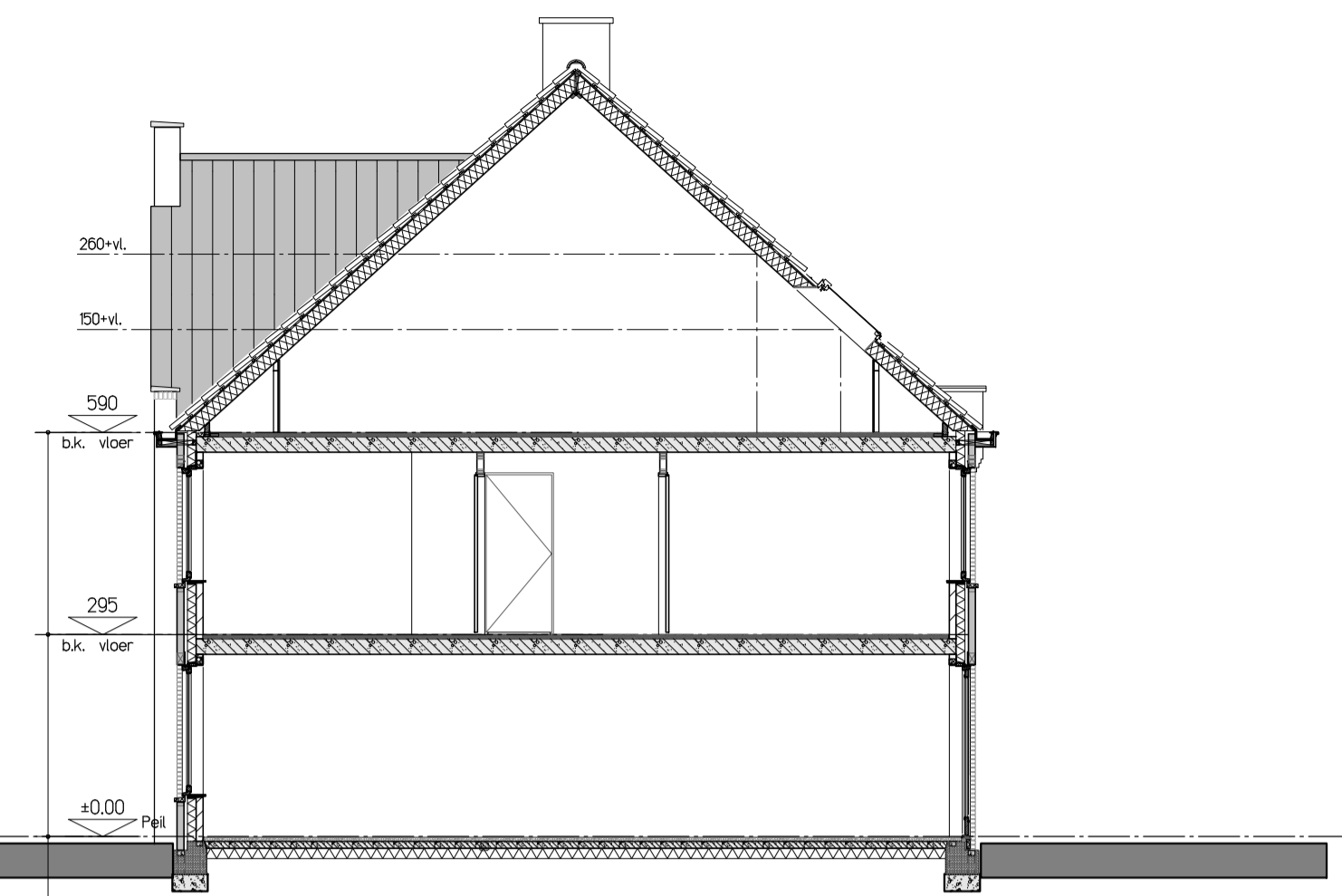
Doorsnede A-A
