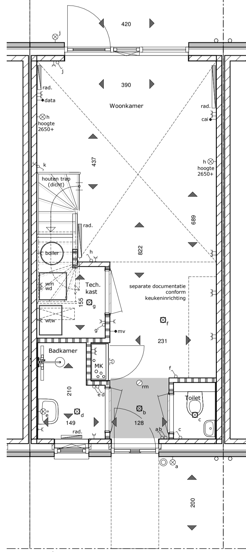
begane grond 1 : 50
