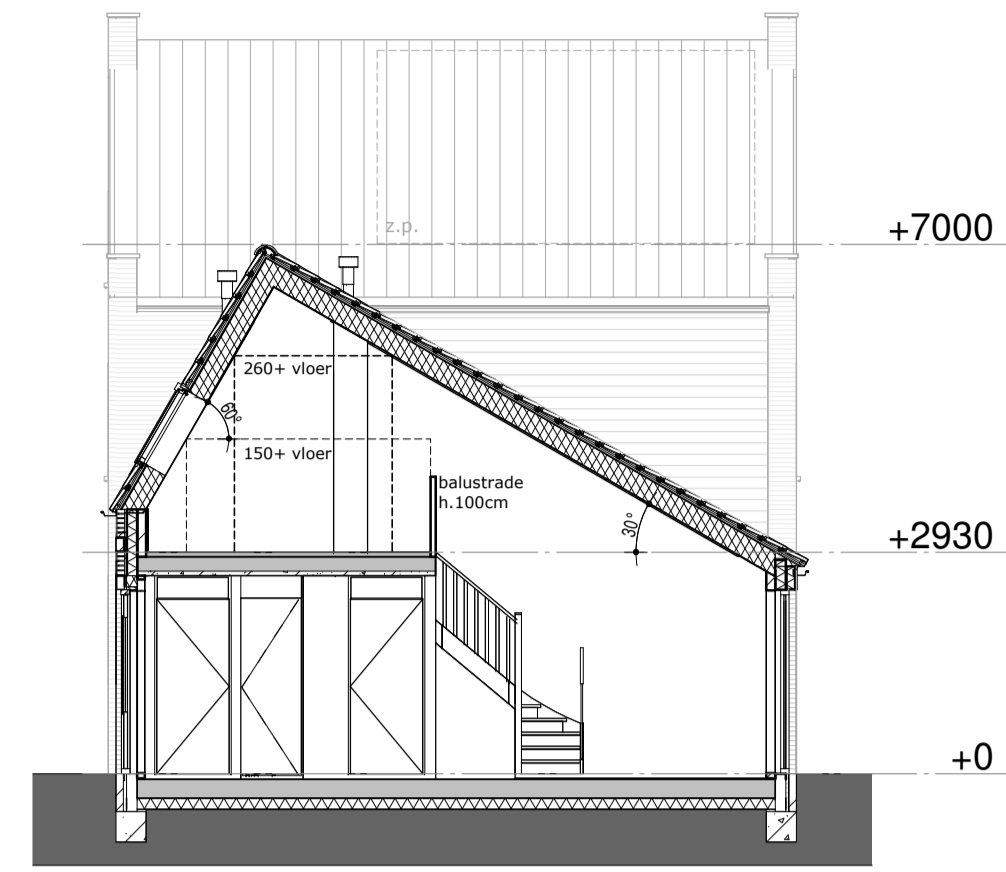
doorsnede 1 : 100
