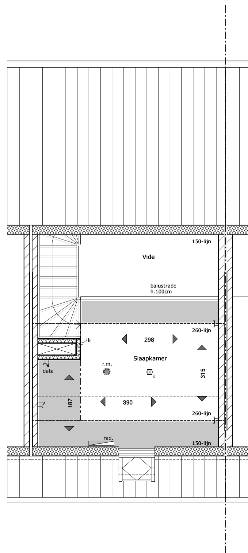
eerste verdieping 1 : 50
