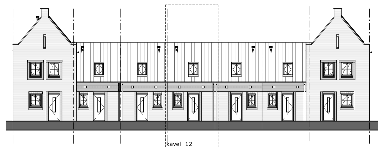
voorgevel
