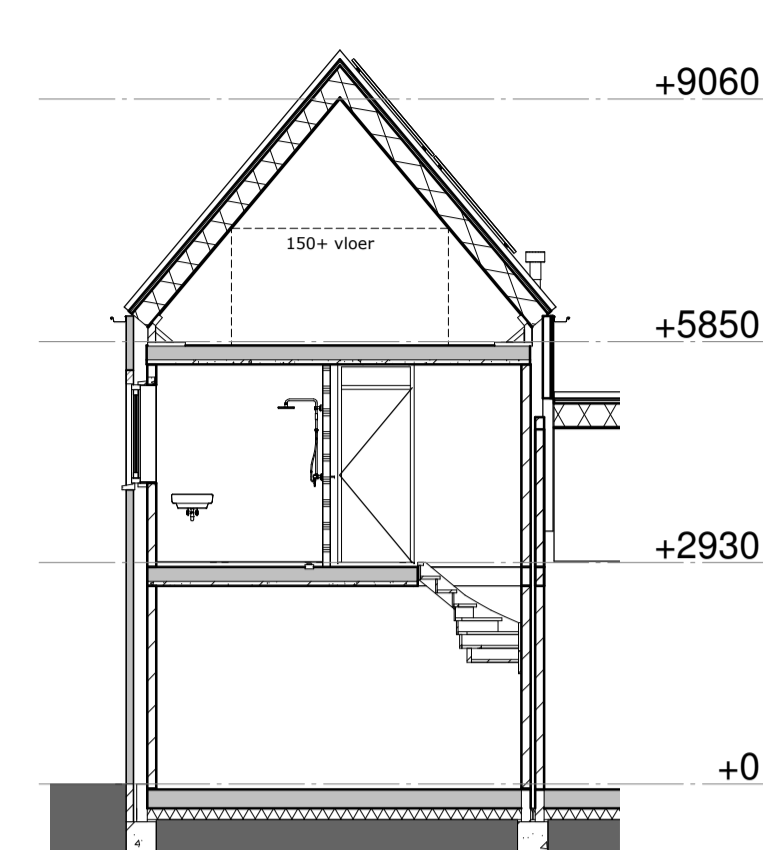
doorsnede 1 : 100
