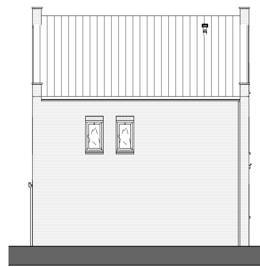
linkergevel 1 : 100
