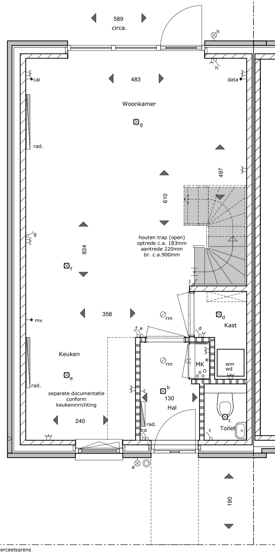
begane grond 1 : 50
