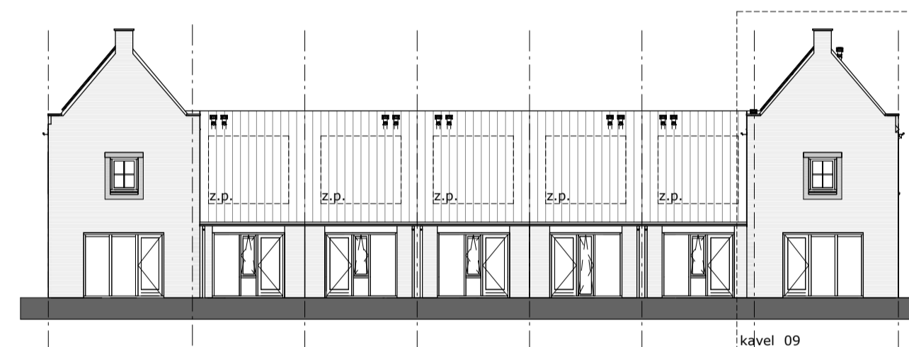
achtergevel
