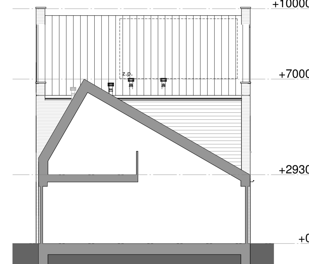
rechtergevel 1 : 100
