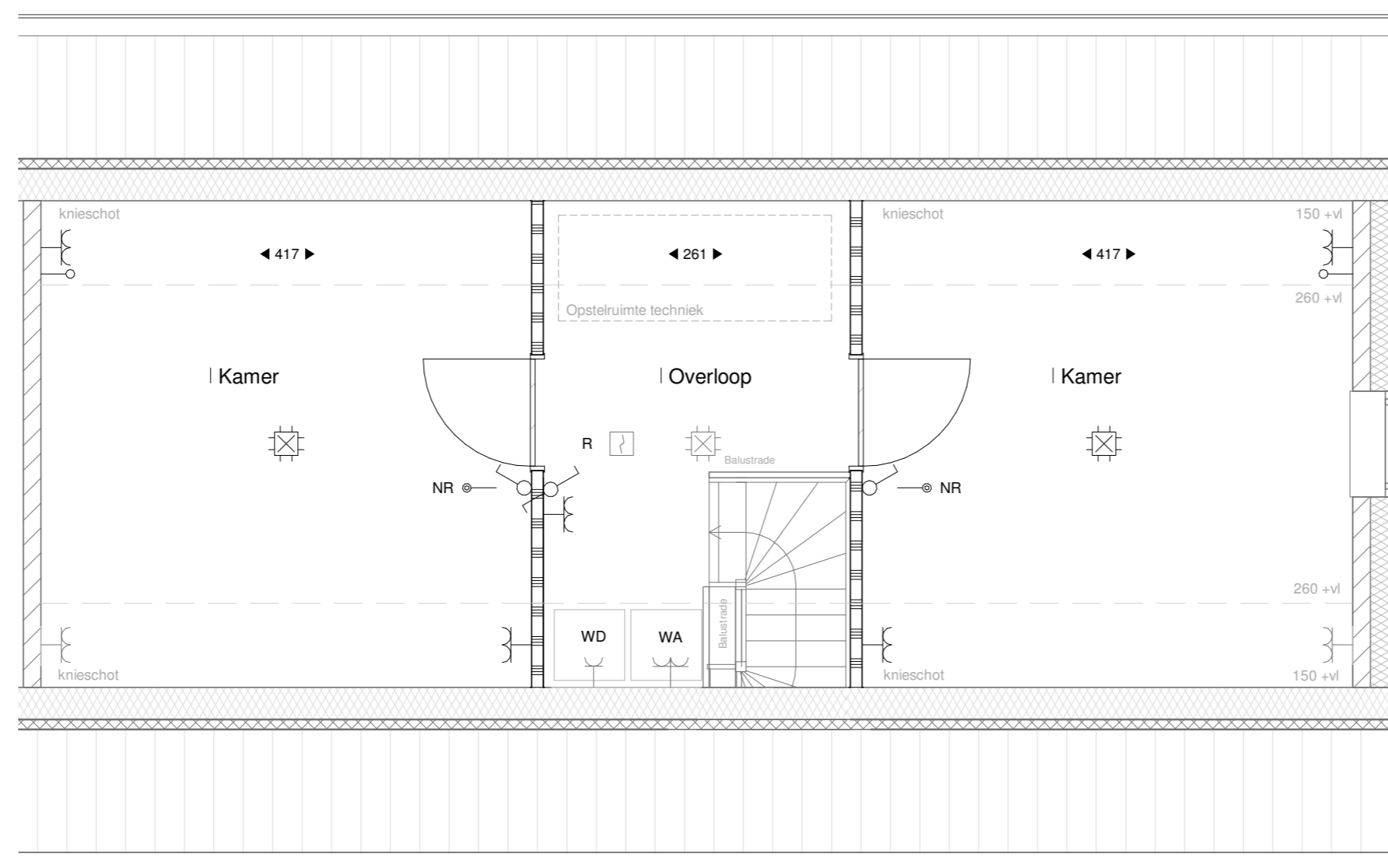
Tweede verdieping 1:50
