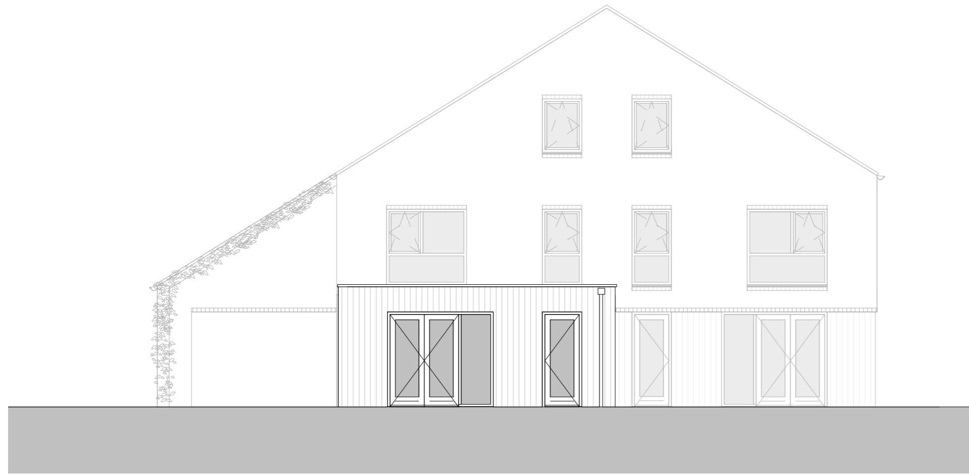
Achtergevel 1 : 100
