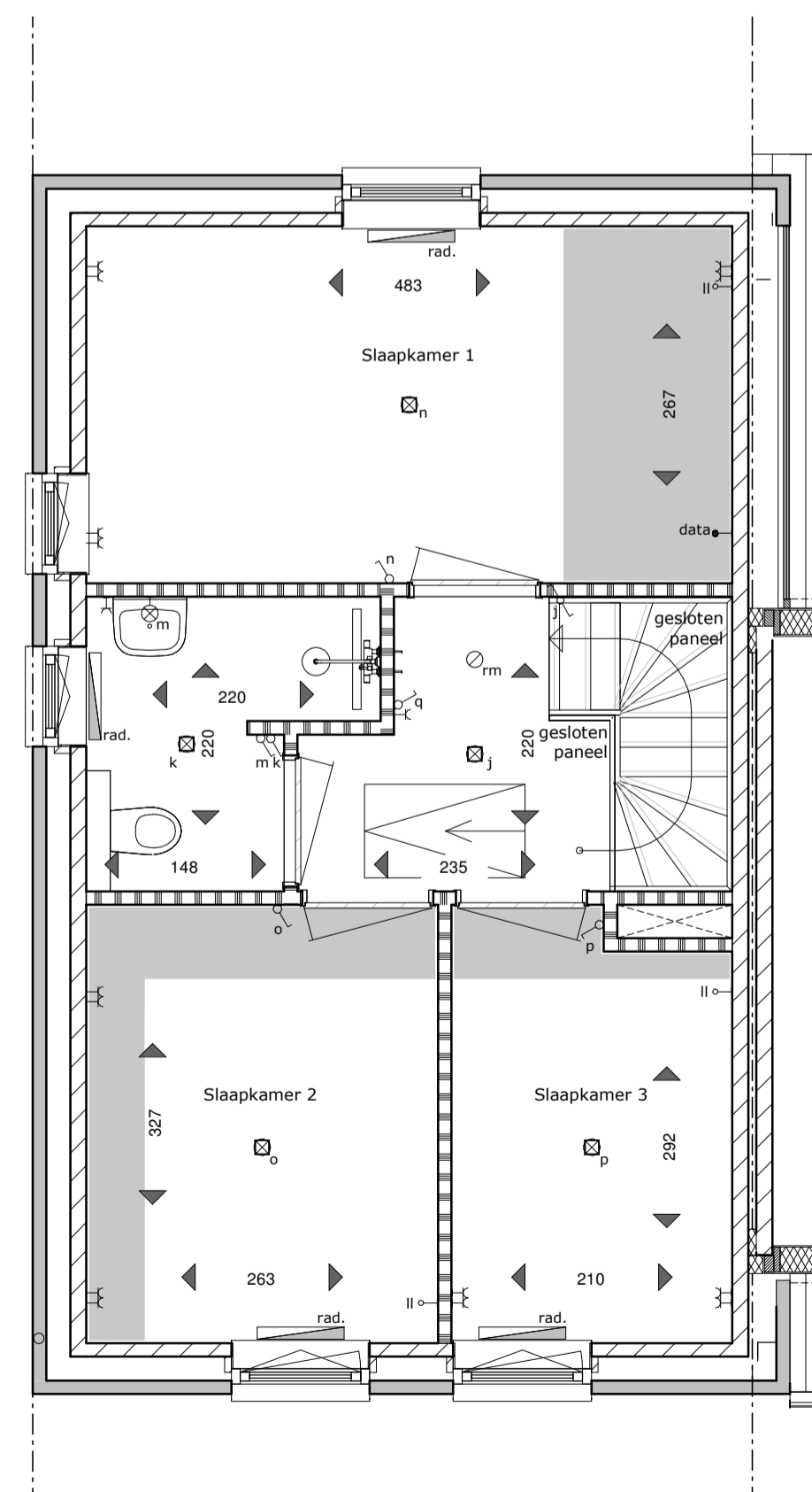
eerste verdieping 1 : 50
