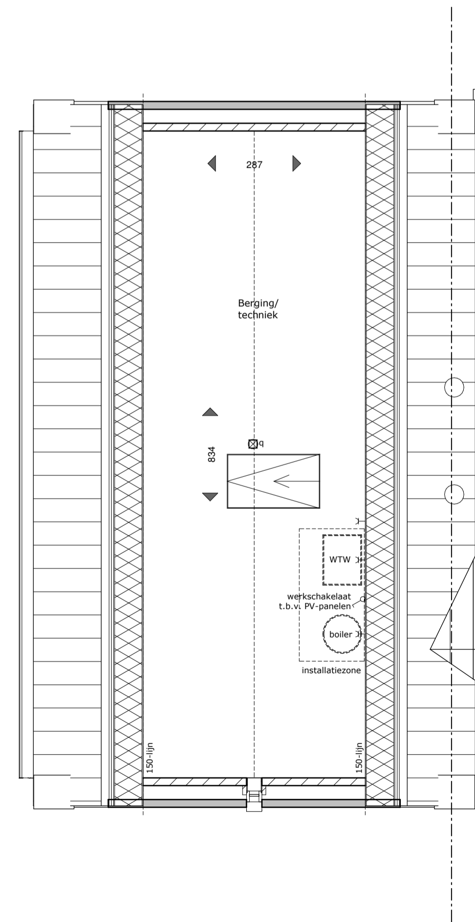
tweede verdieping 1 : 50
