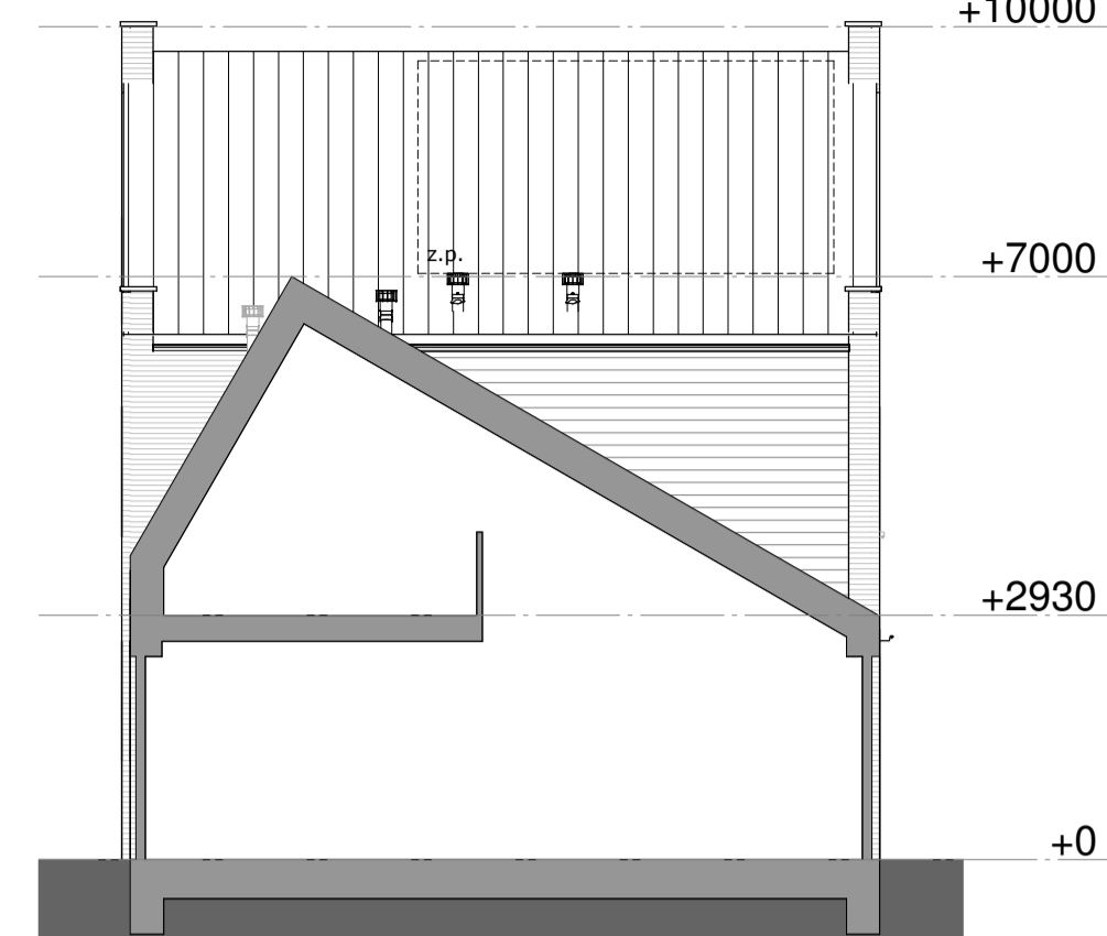
rechtergevel 1 : 100
