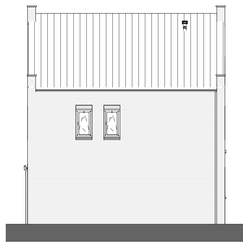
linkergevel 1 : 100
