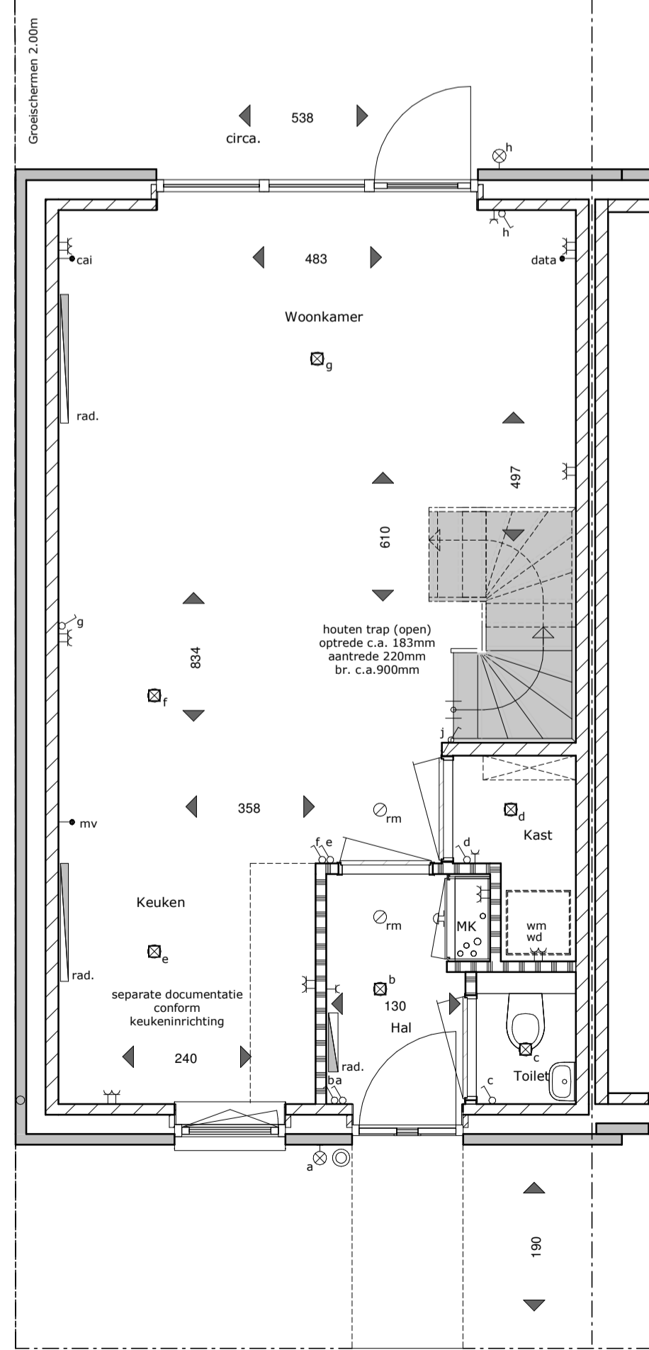
begane grond 1 : 50
