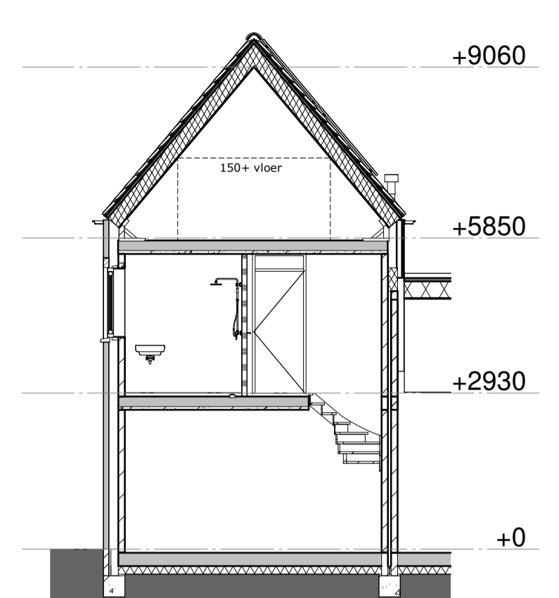
doorsnede 1 : 100
