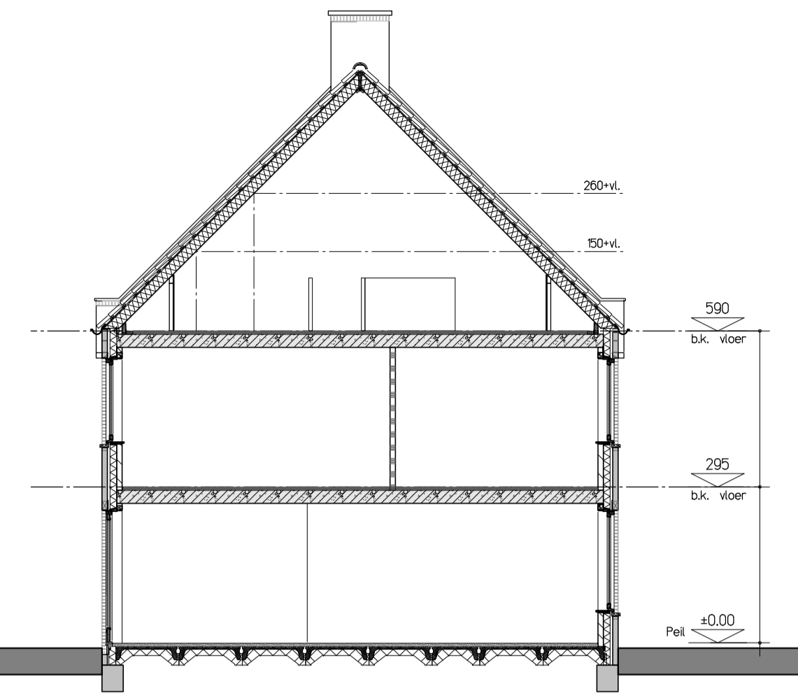
Doorsnede A-A
