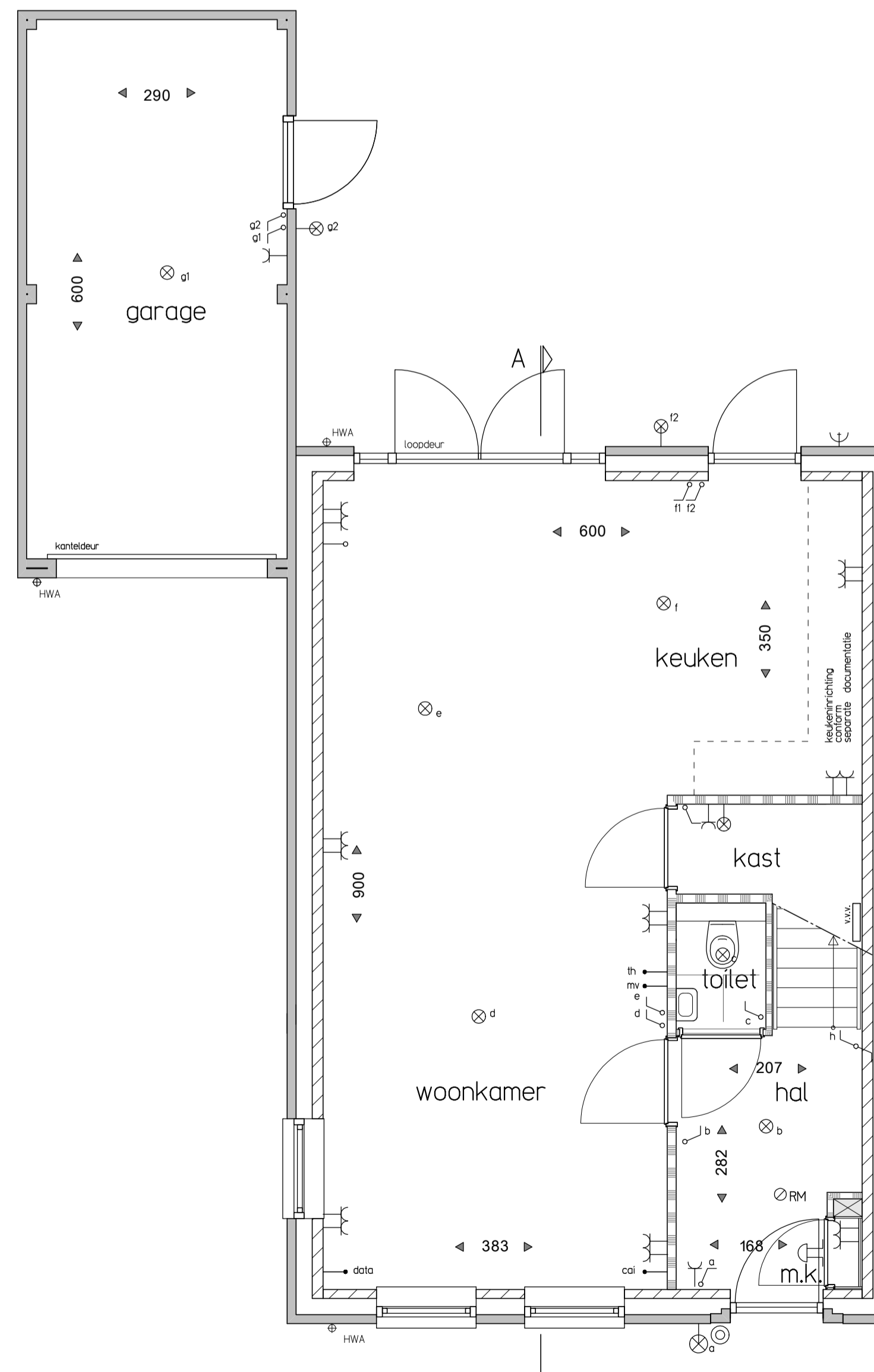
Begane grond
