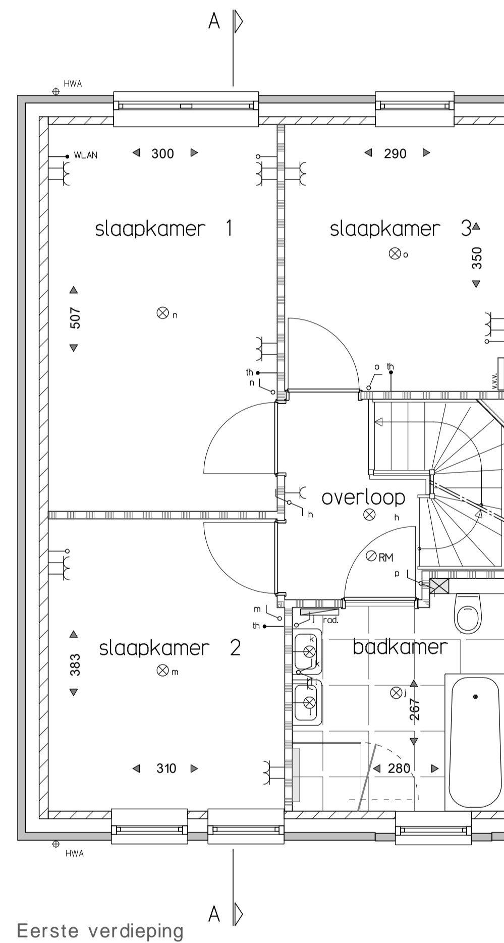
Eerste verdieping
