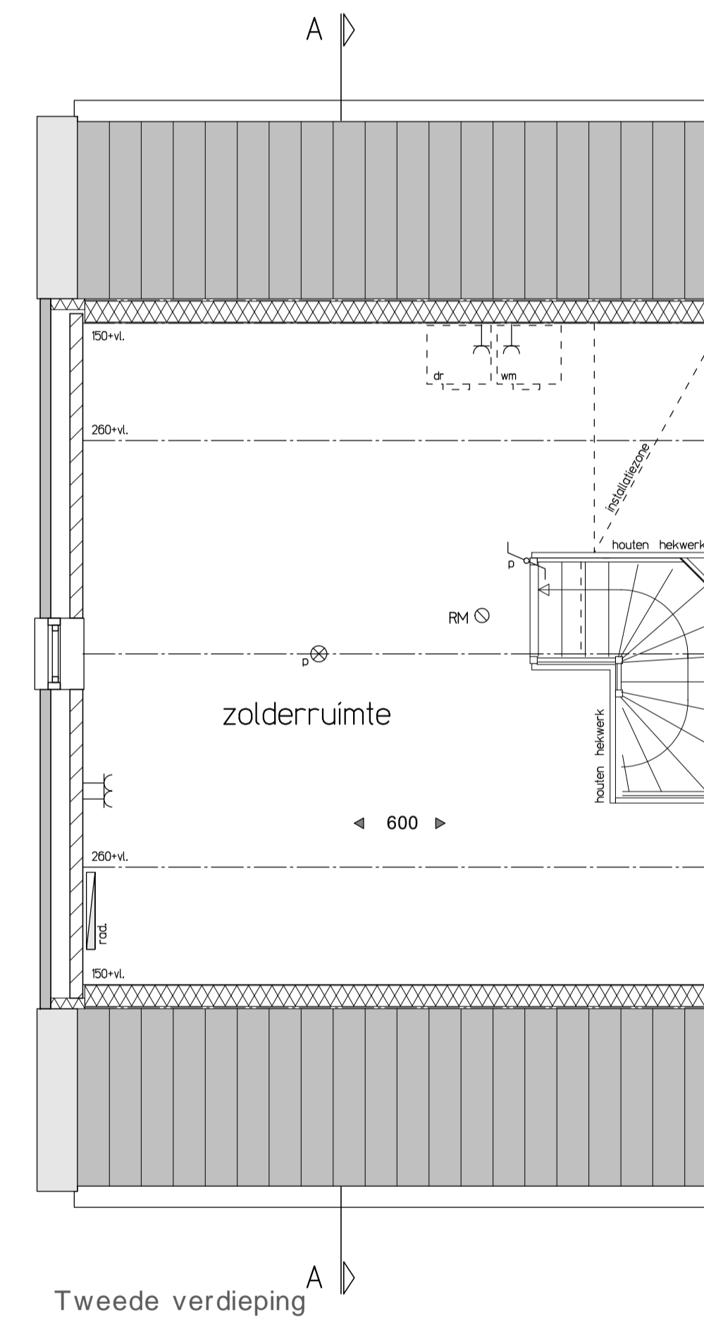
Tweede verdieping
