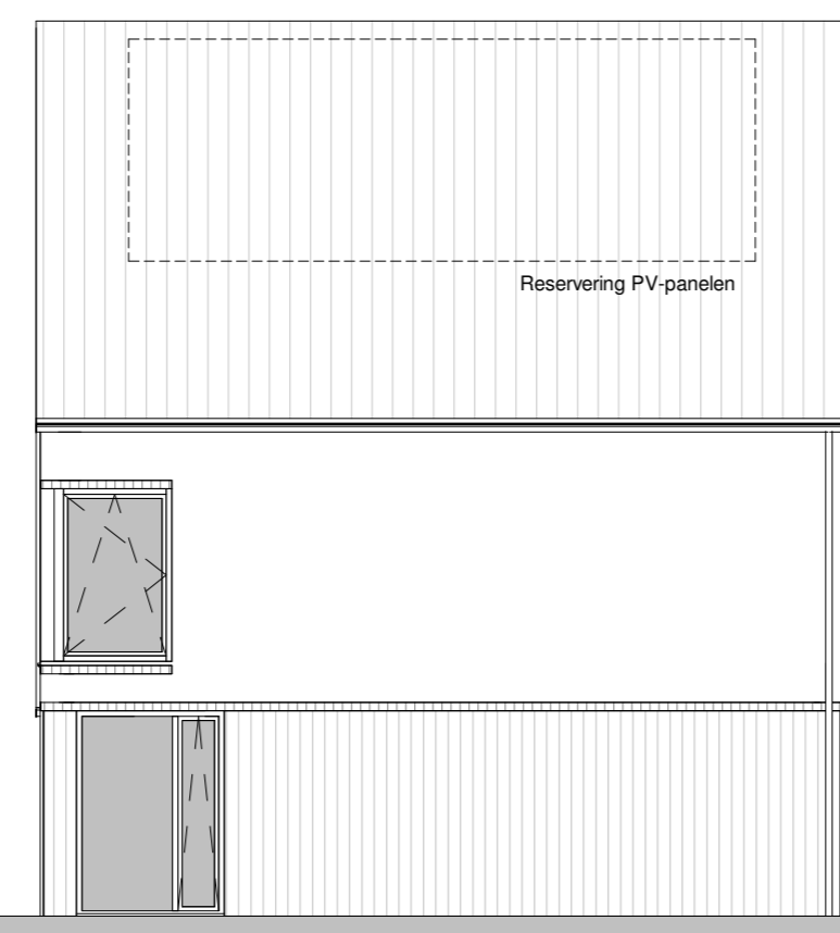
Rechterzijgevel 1:100
