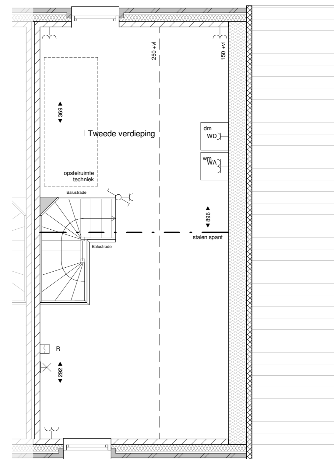
Tweede verdieping 1:50
