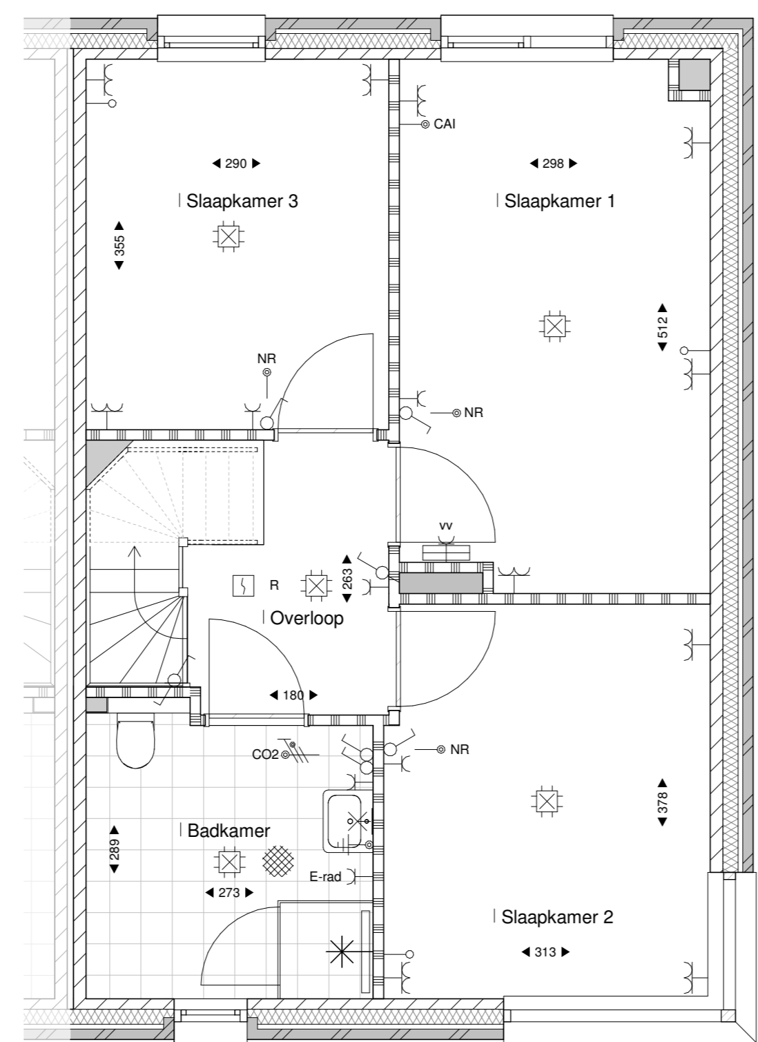
Eerste verdieping 1:50
