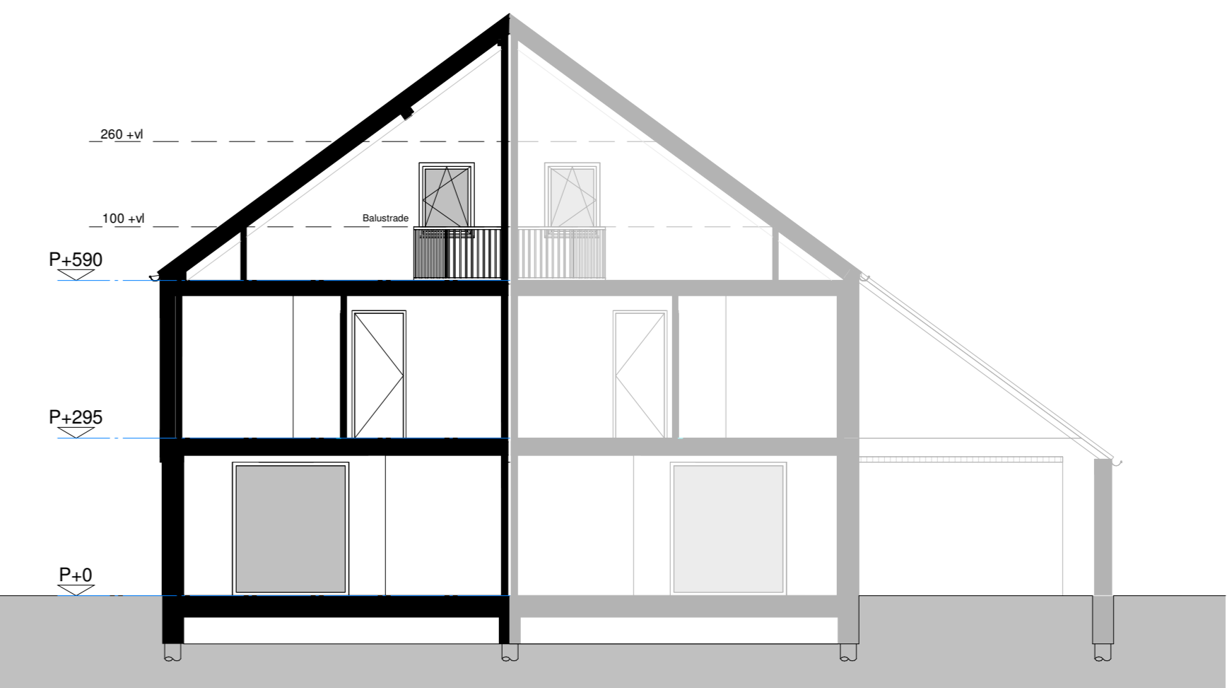
Doorsnede AA 1:100
