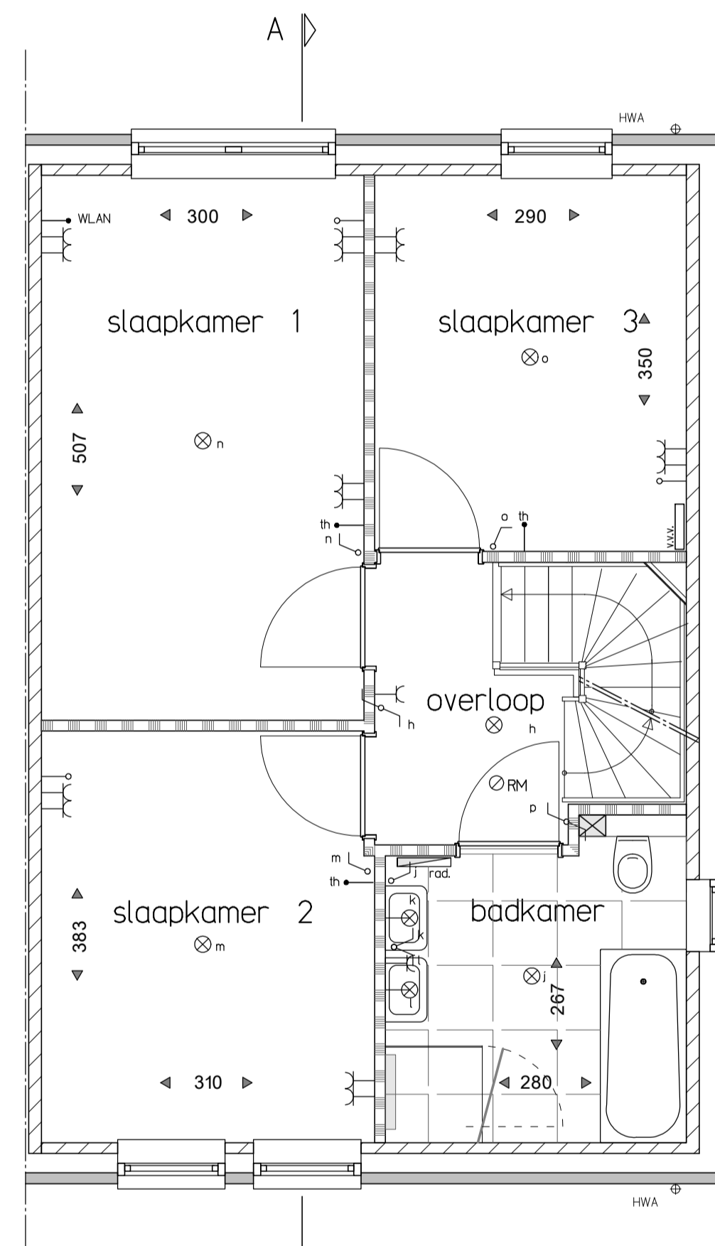
Eerste verdieping
