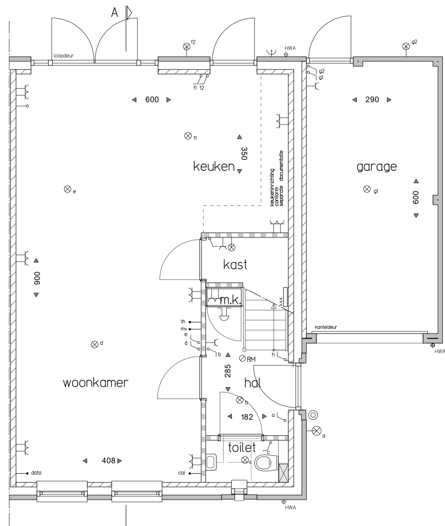
Begane grond
