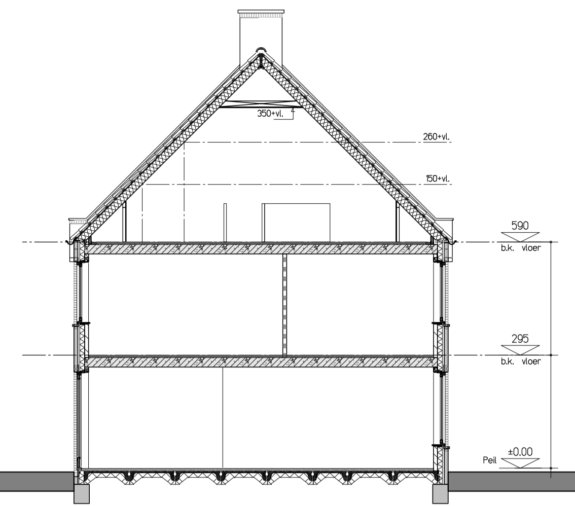
Doorsnede A-A
