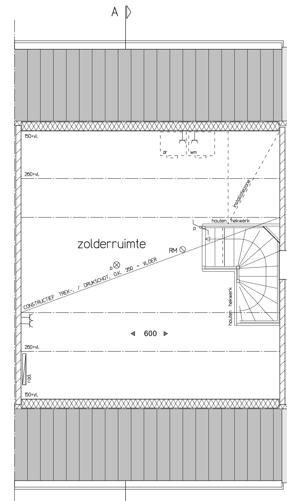
Tweede verdieping
