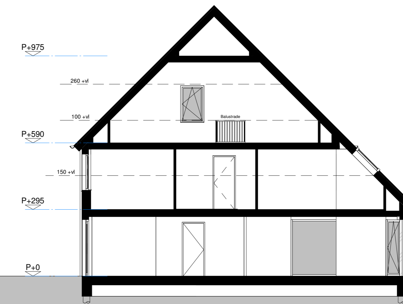
Doorsnede BB 1:100
