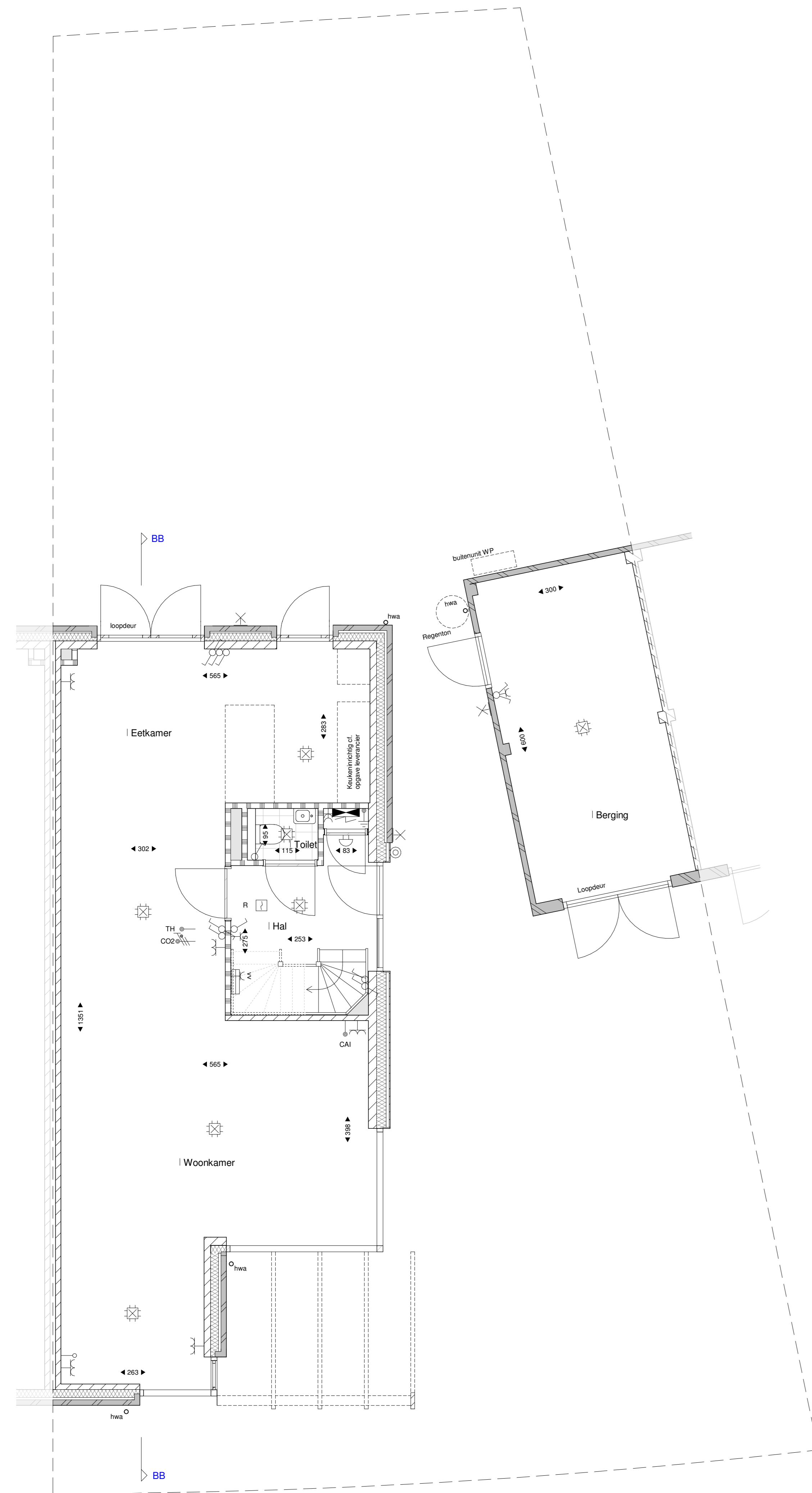
Begane grond 1:100
