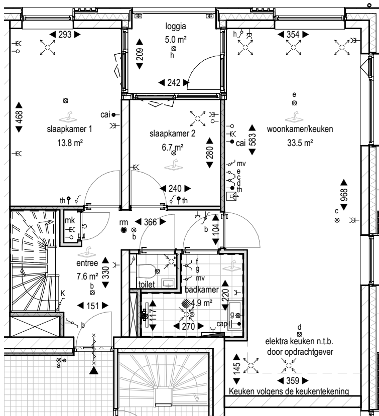
plaattegrond woonlaag 1
