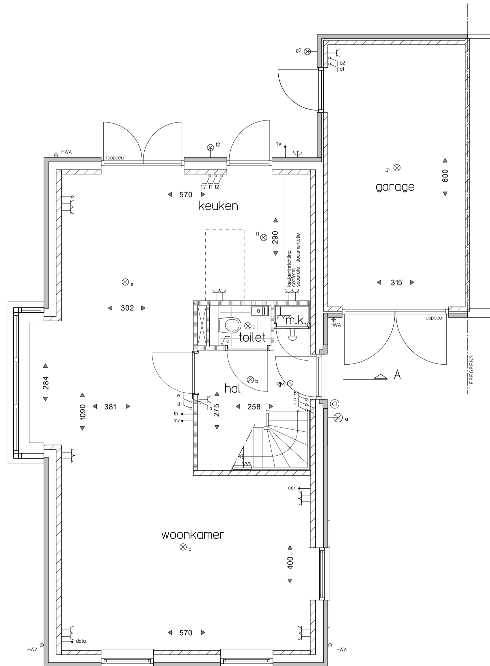
Begane grond
