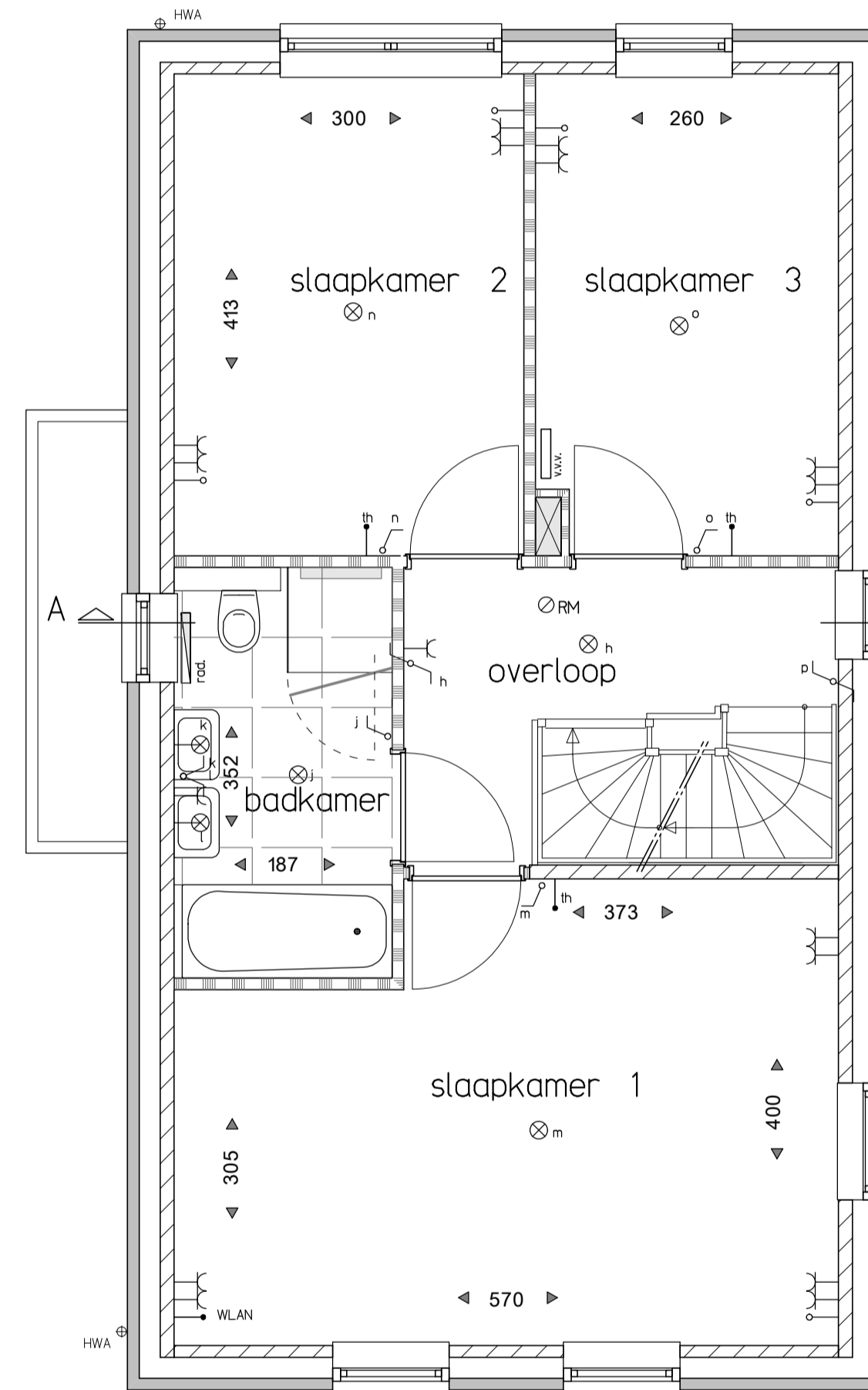
Eerste verdieping
