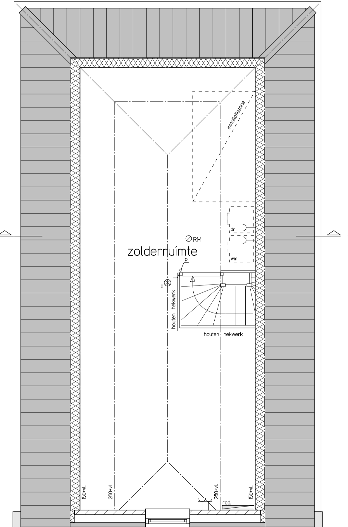
Tweede verdieping
