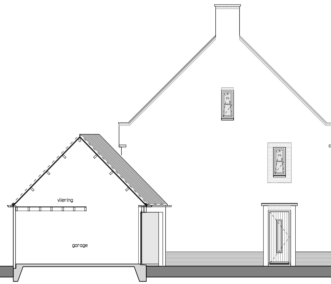
Doorsnede garage
