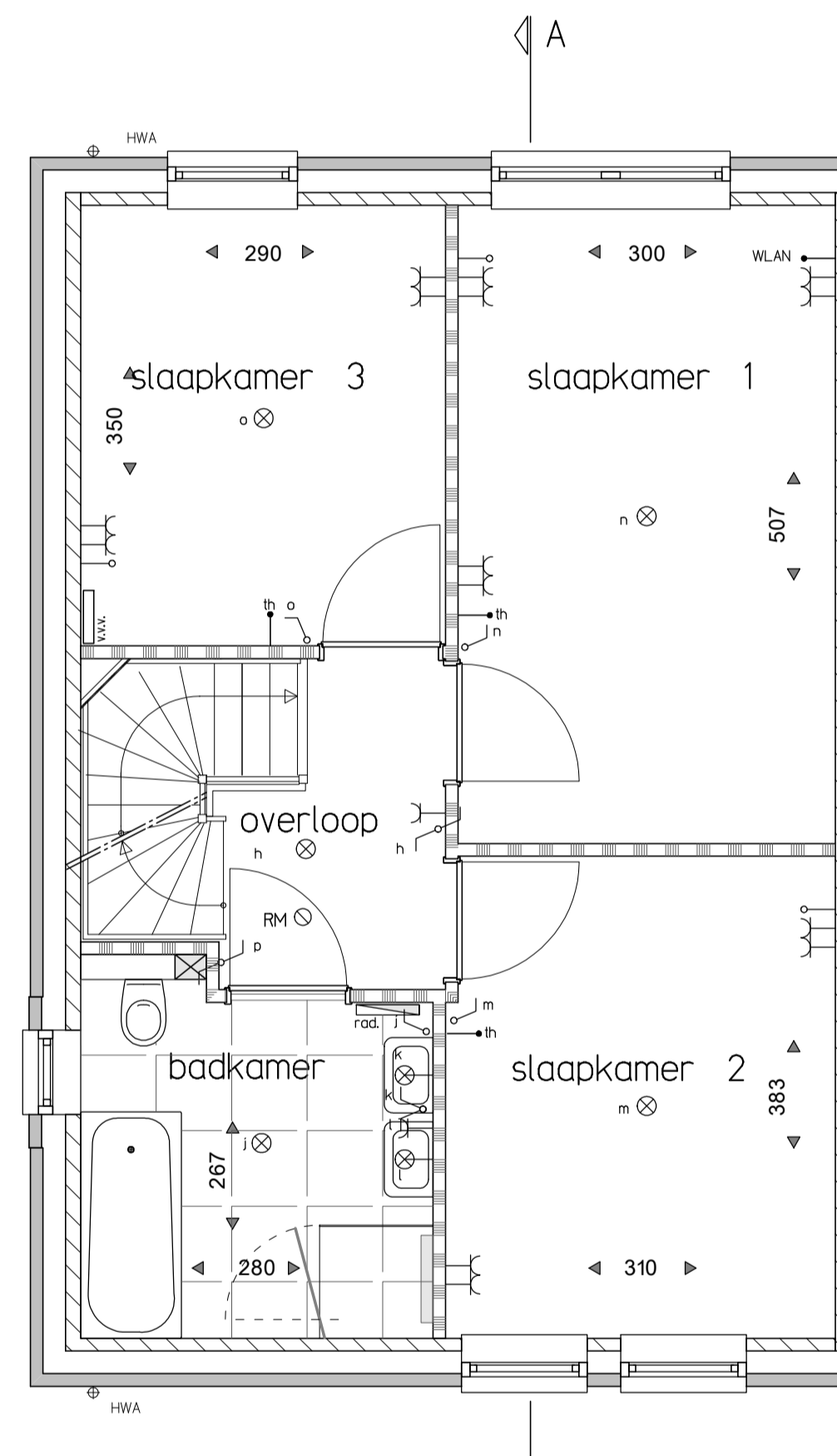
Eerste verdieping
