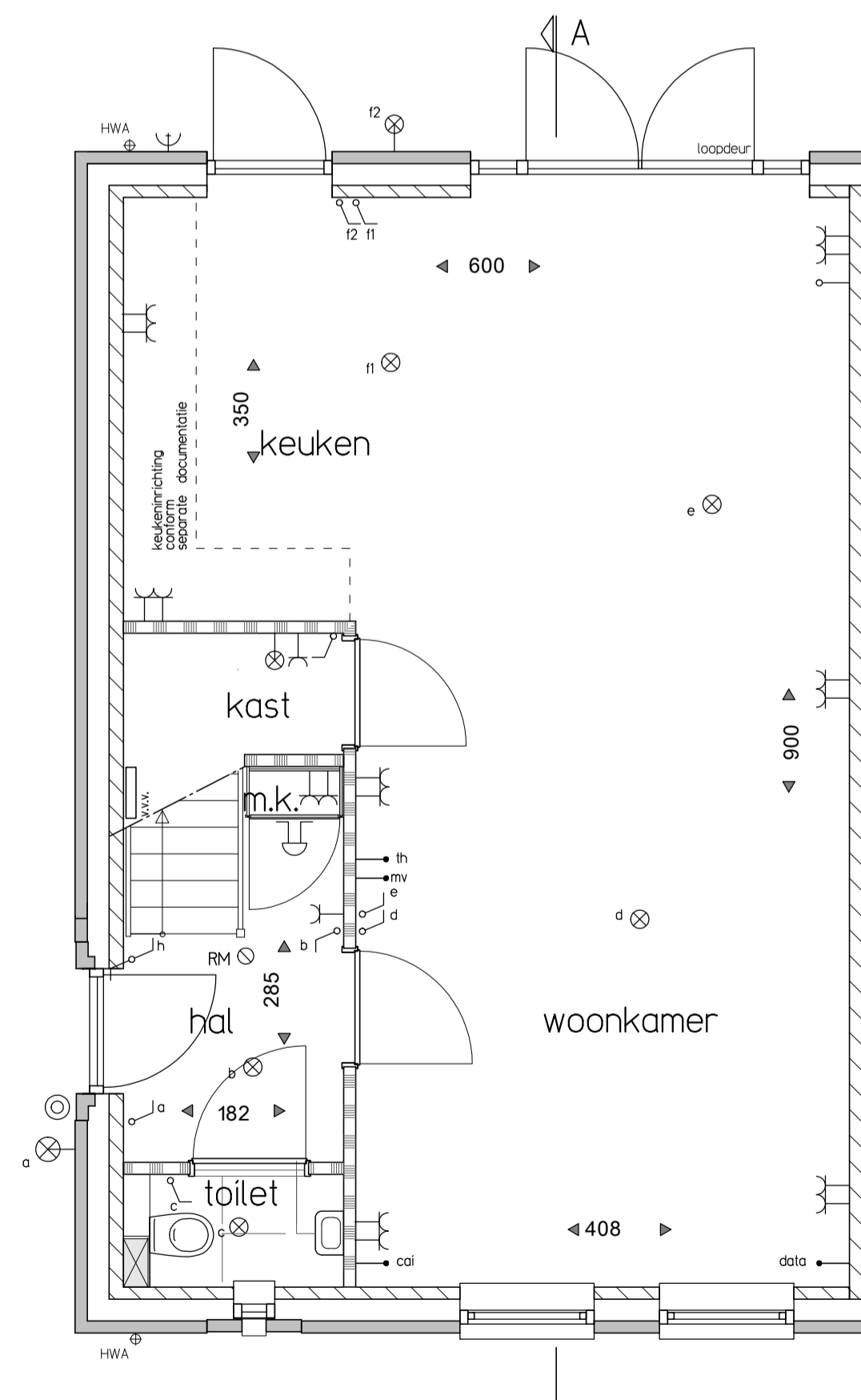
Begane grond
