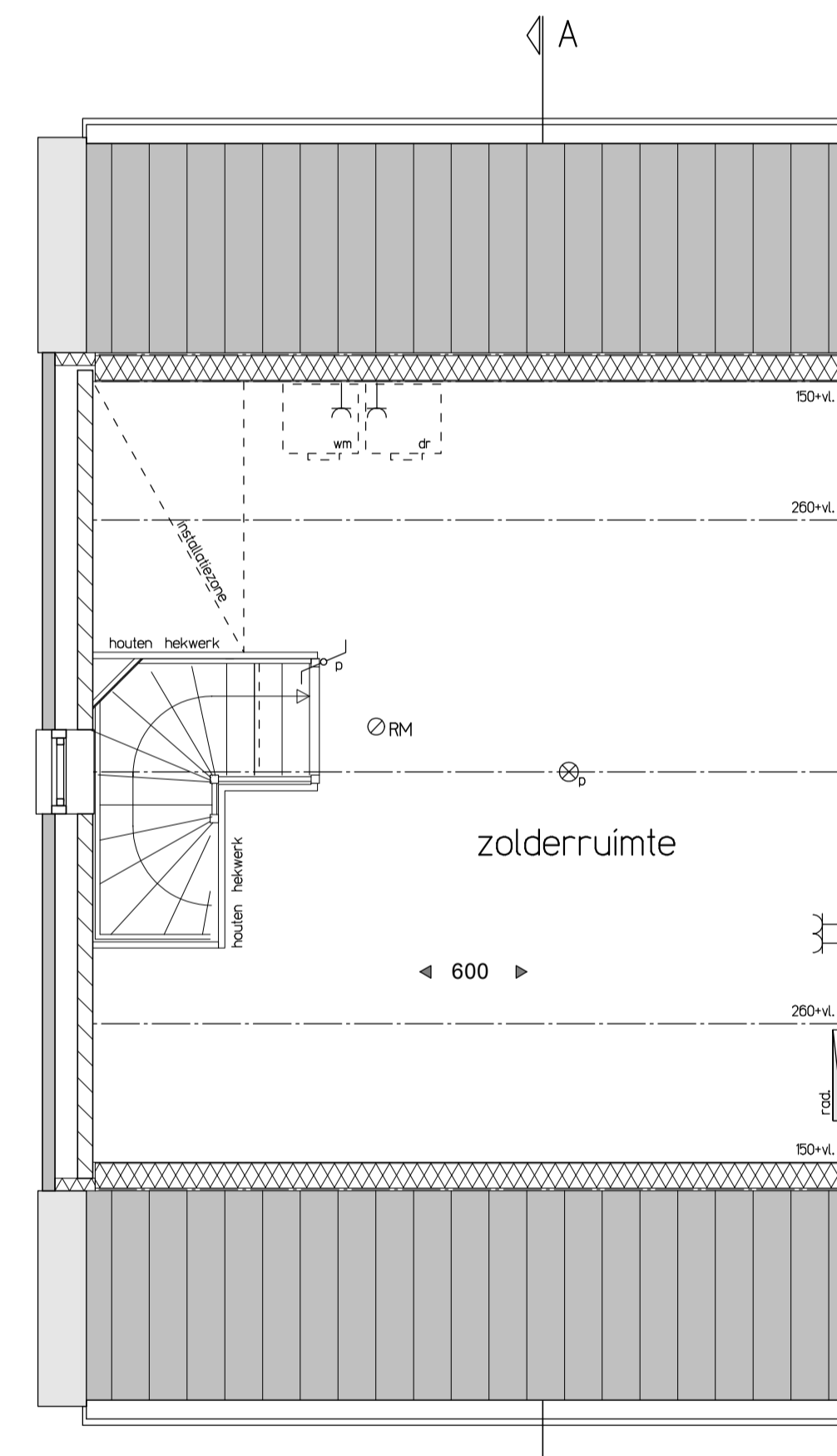
Tweede verdieping
