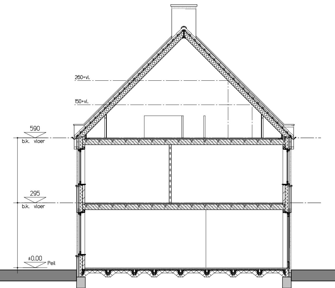
Doorsnede A-A
