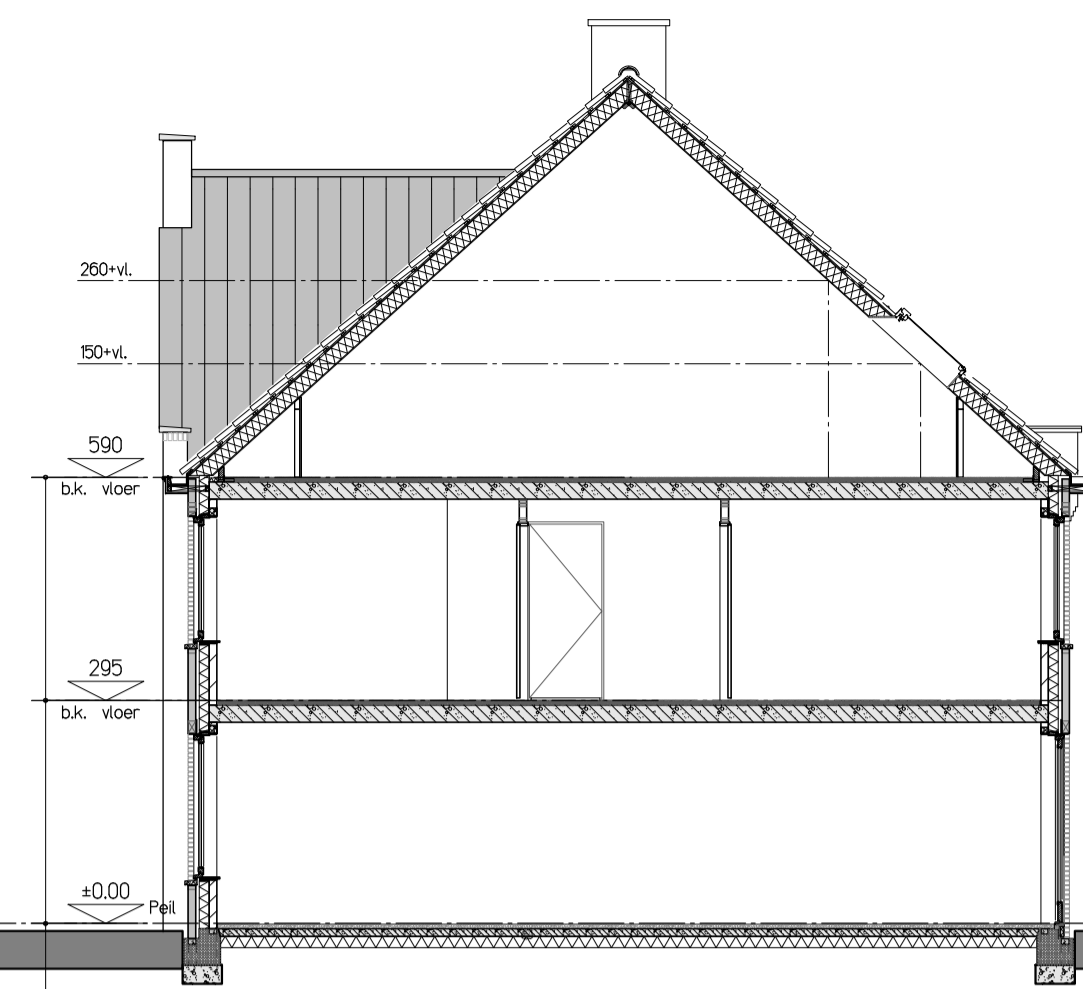
Doorsnede A-A
