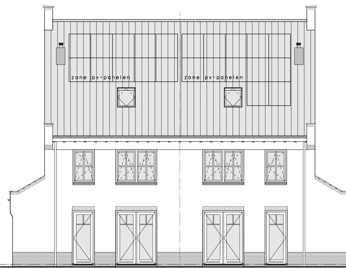
Achtergevel Type D
