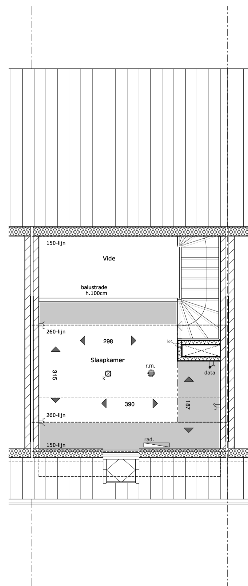
eerste verdieping 1 : 50
