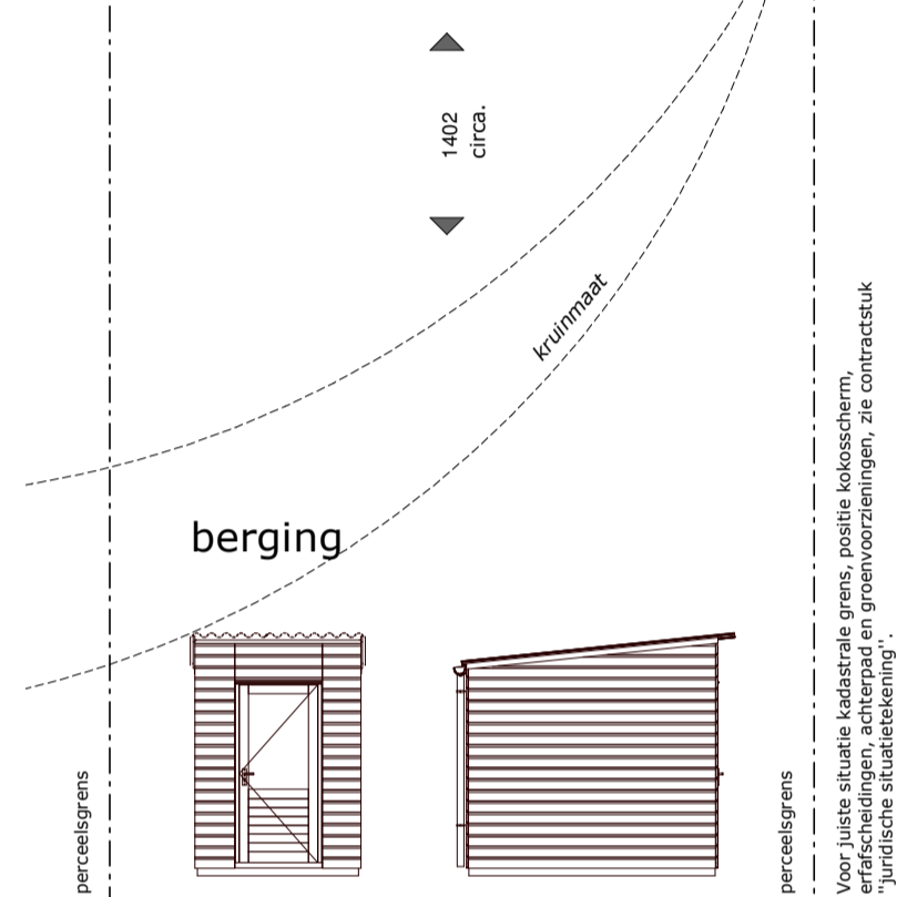
voor- en zijaanzicht 1 : 100
