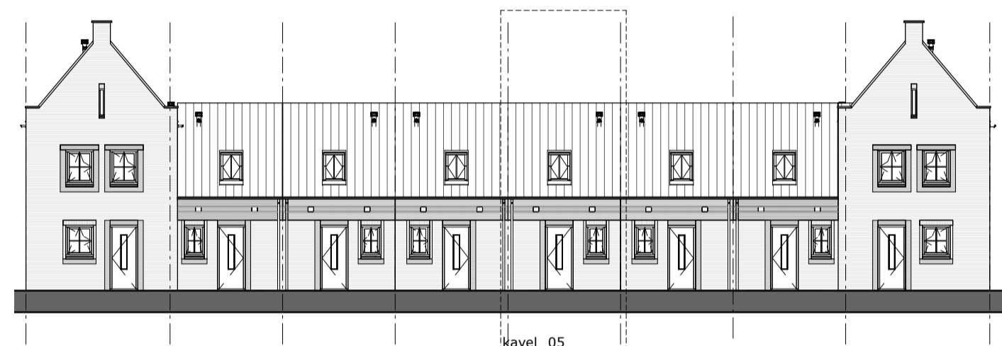
voorgevel
