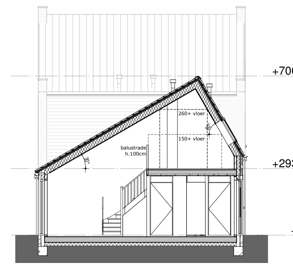
doorsnede 1 : 100
