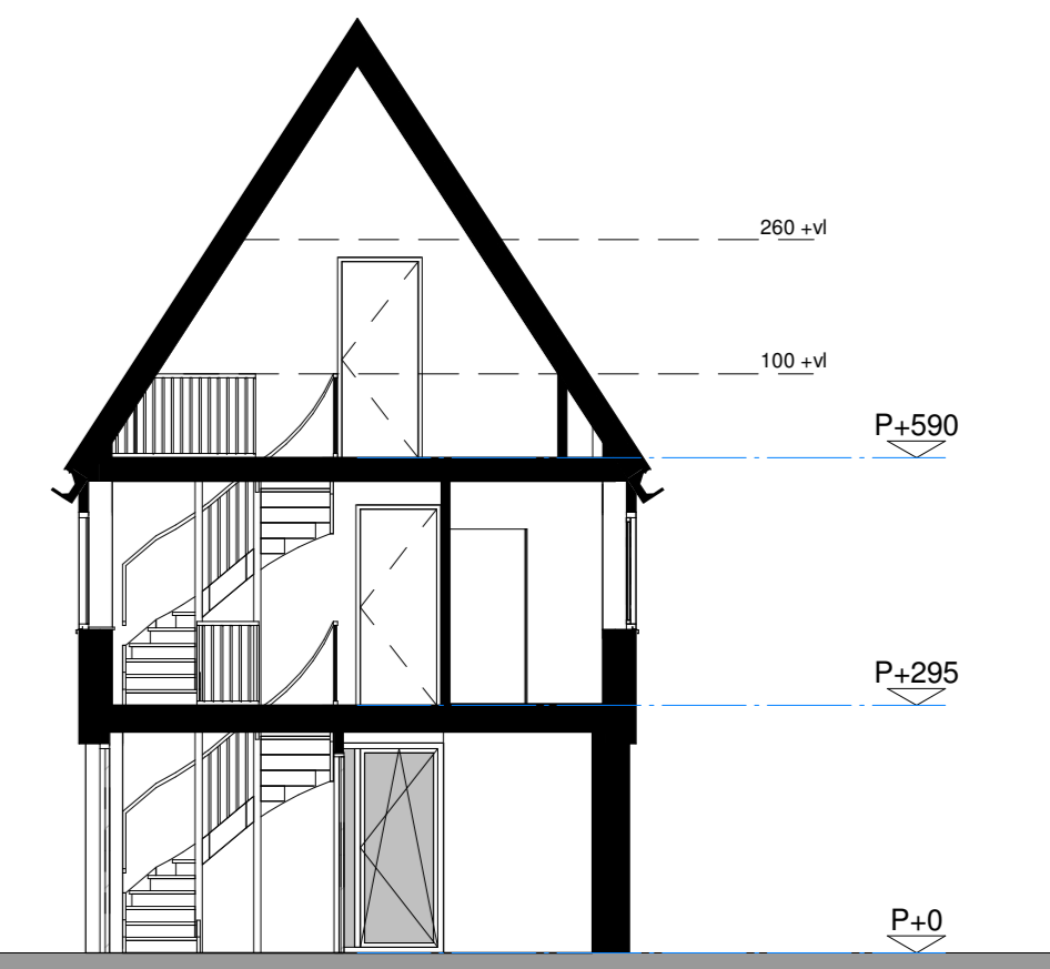
Doorsnede AA 1:100
