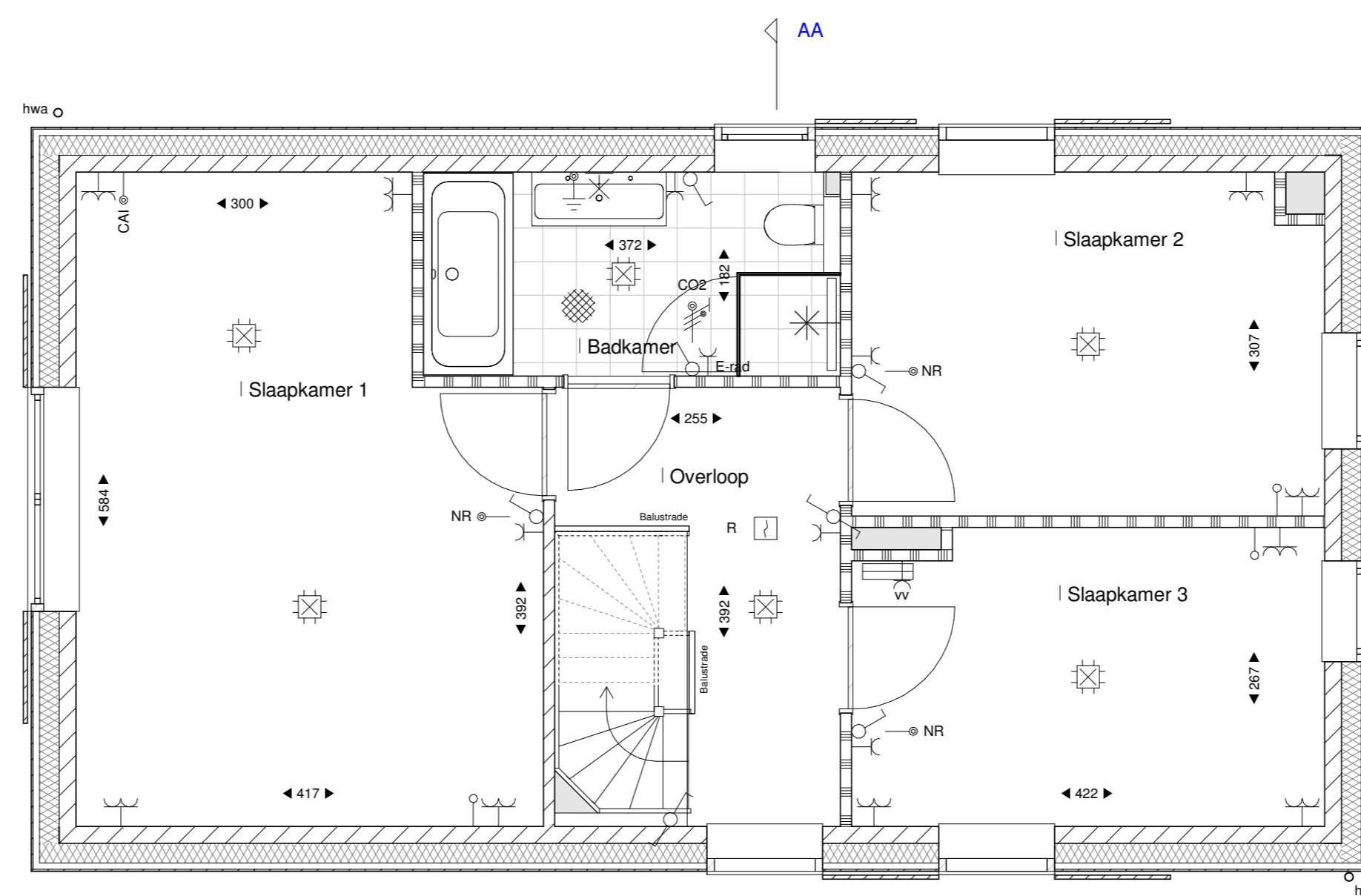
Eerste verdieping 1:100
