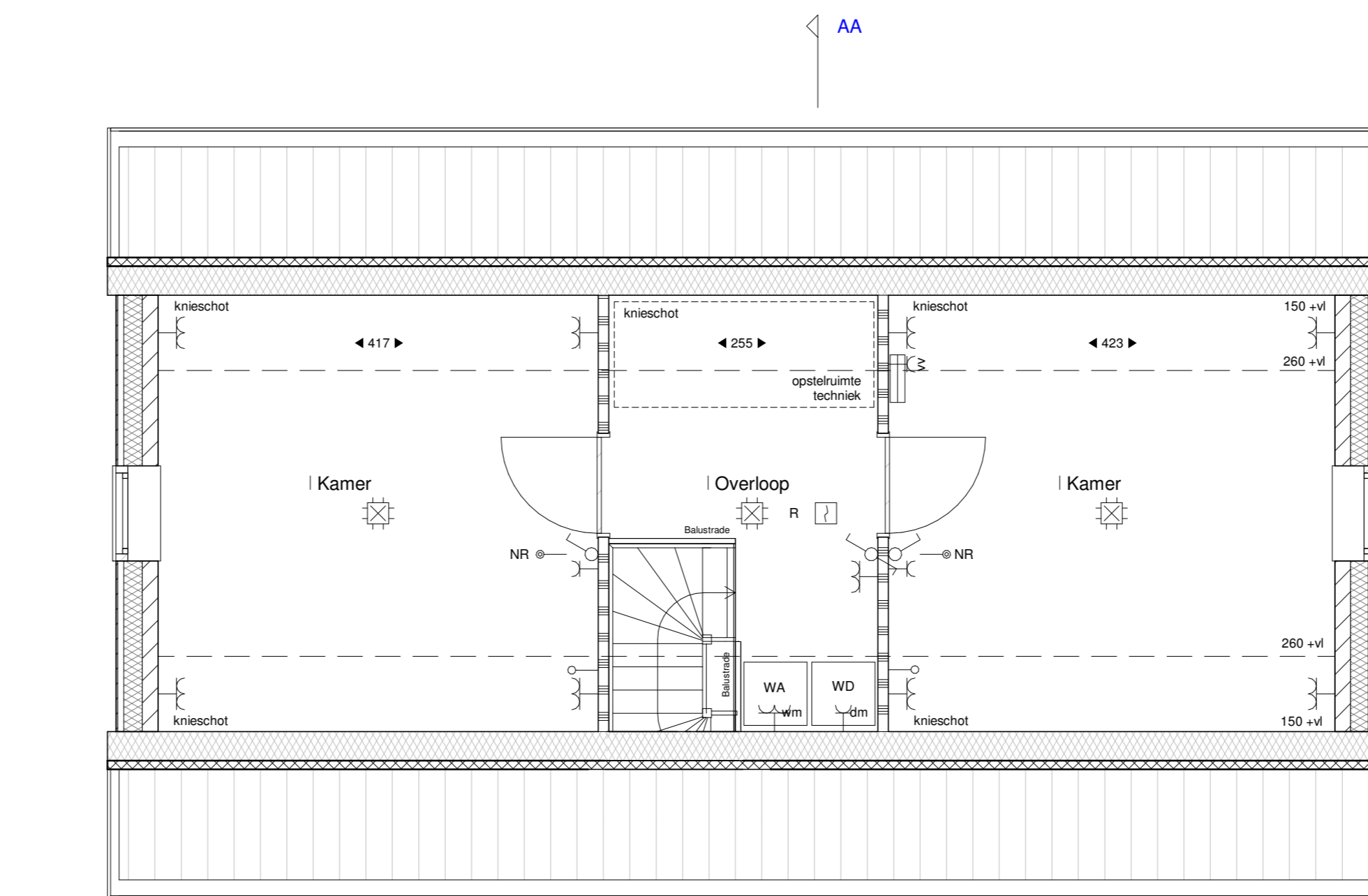
Tweede verdieping 1:100
