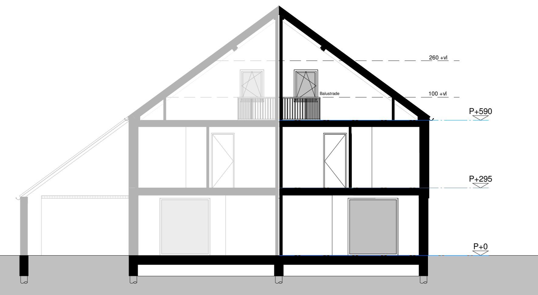
Doorsnede 1:100
