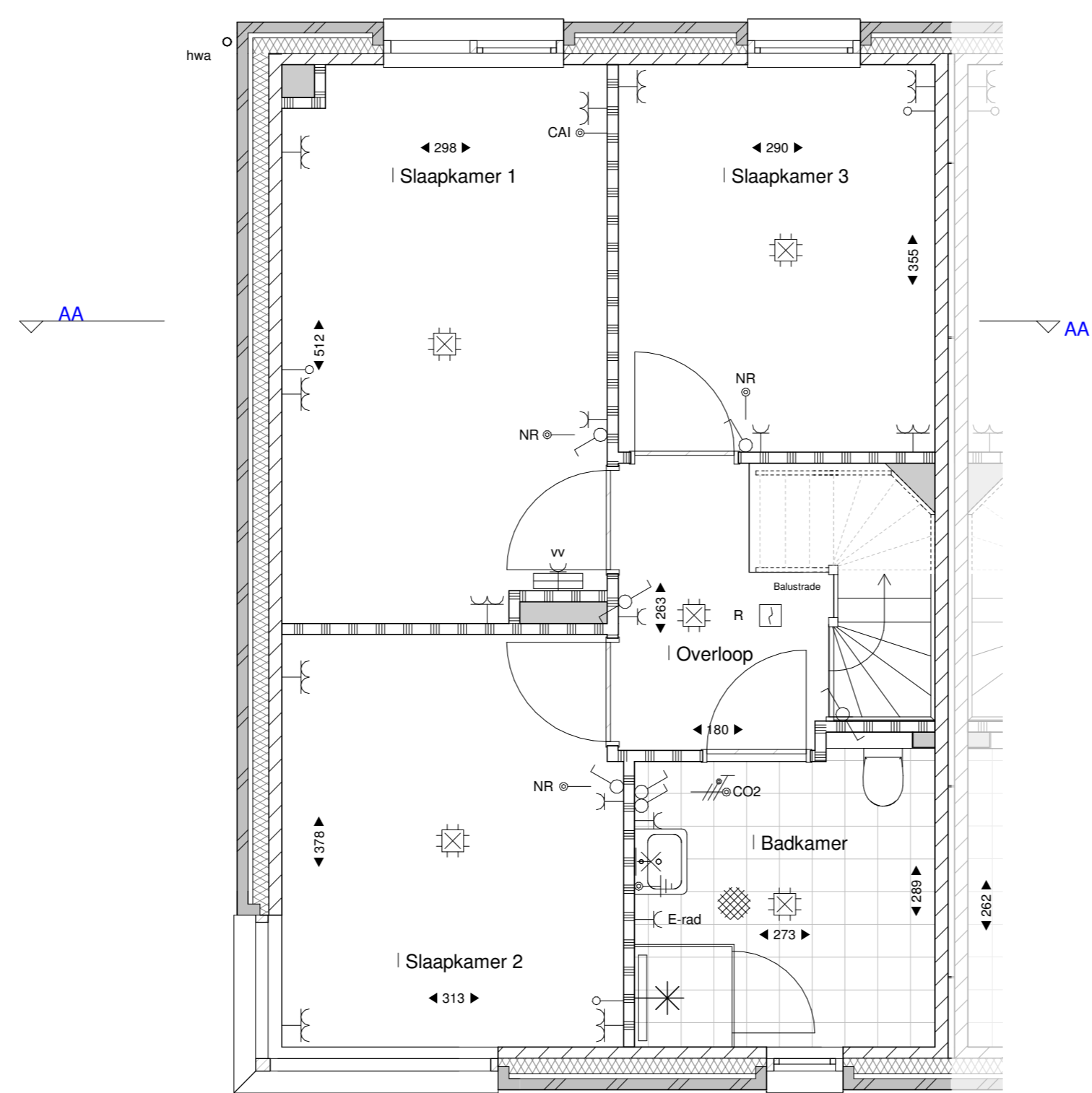
Eerste verdieping 1:50
