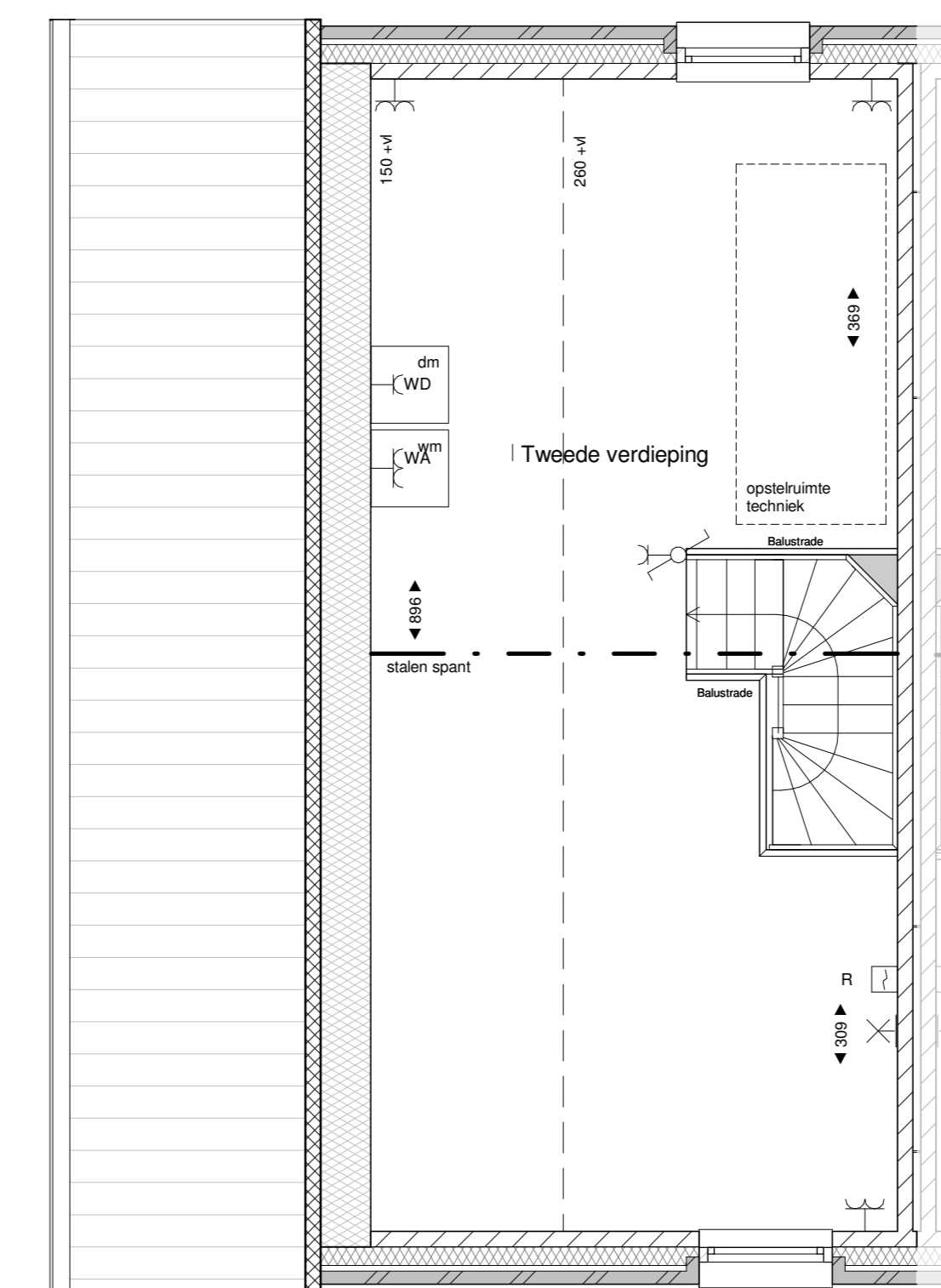
Tweede verdieping 1:50
