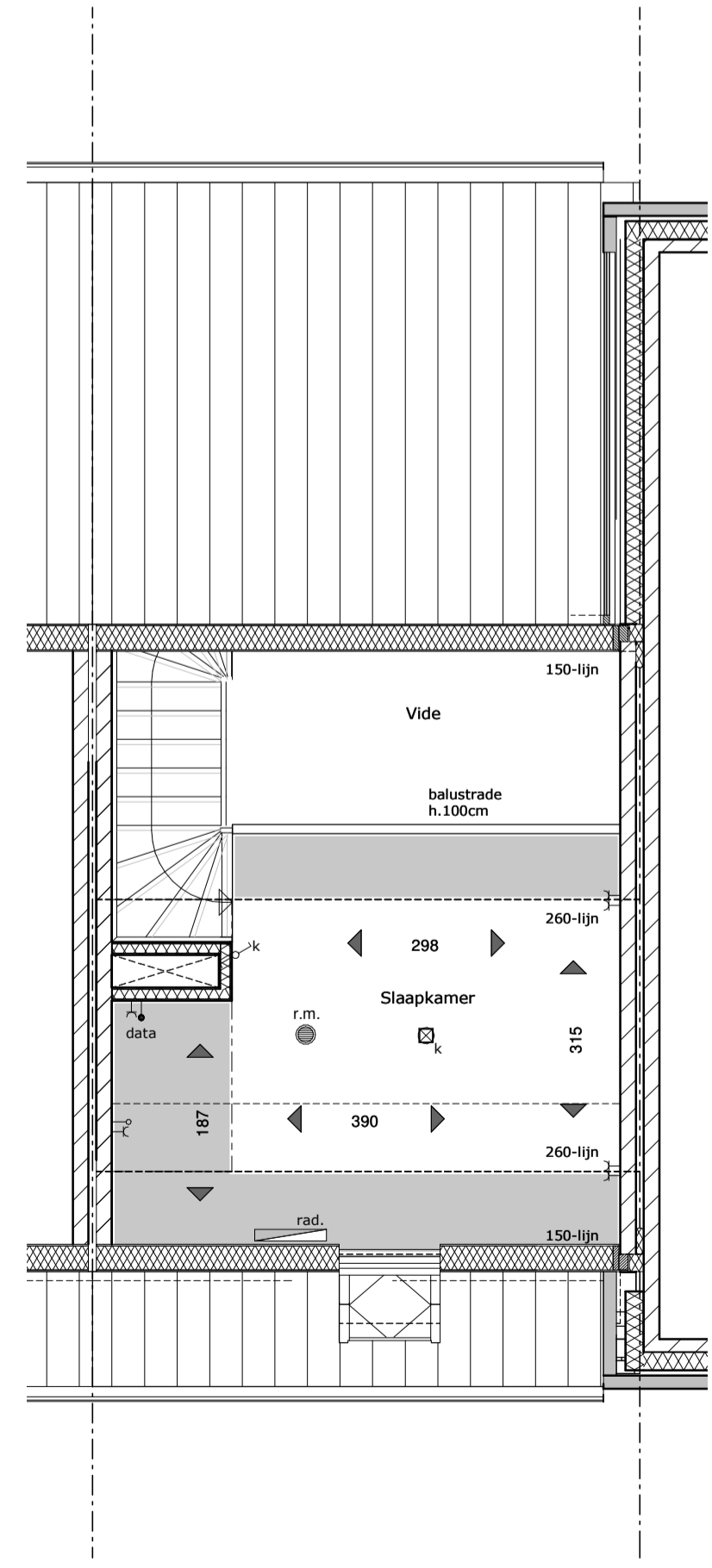
eerste verdieping 1 : 50
