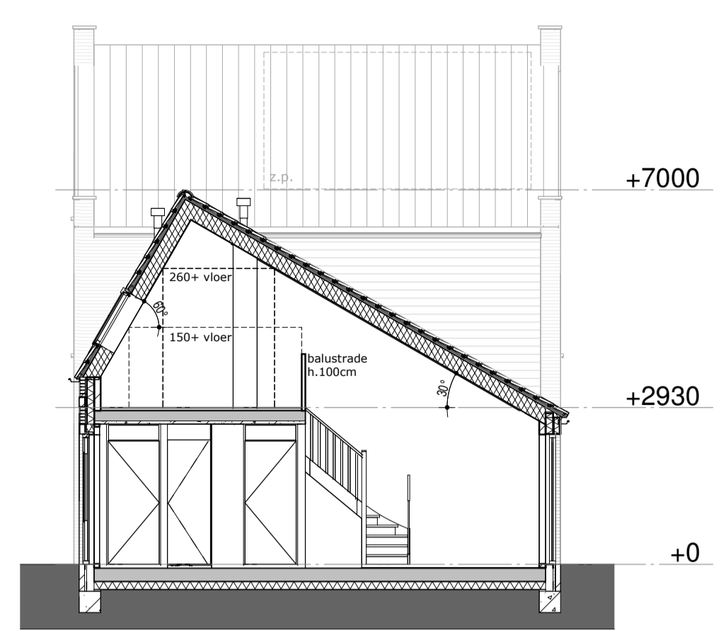
doorsnede 1 : 100
