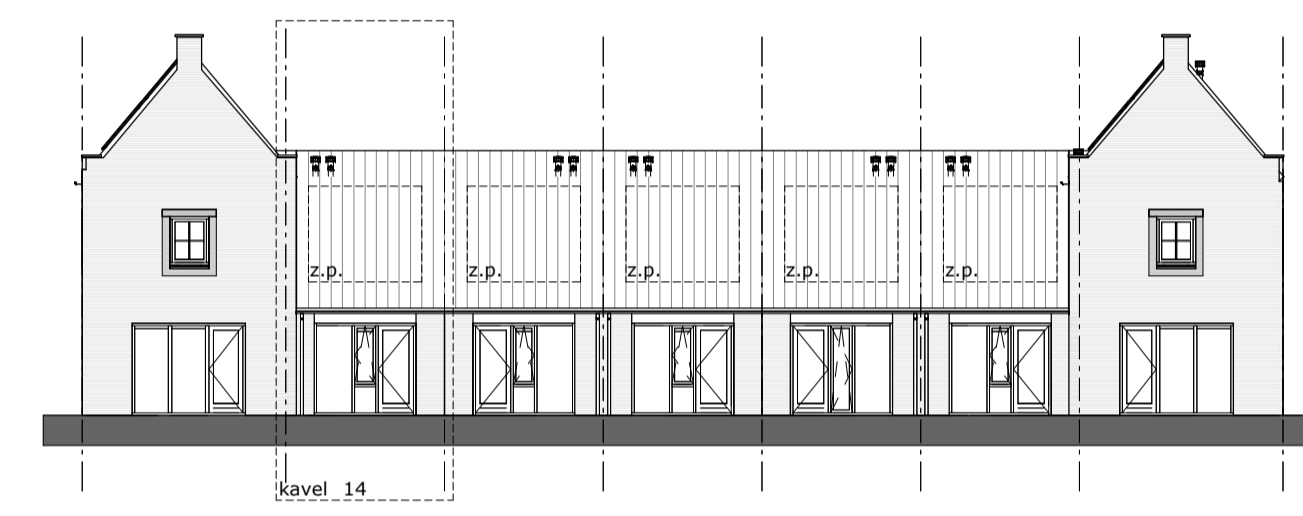
achtergevel
