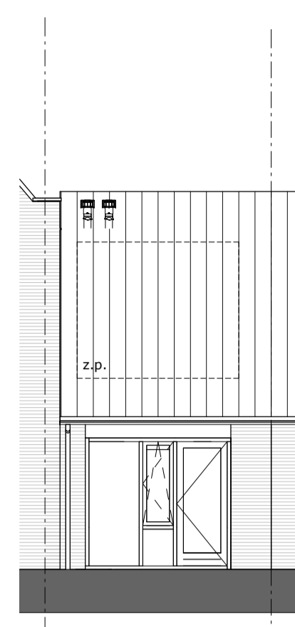
achtergevel 1 : 100
