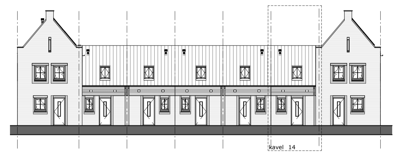
voorgevel
