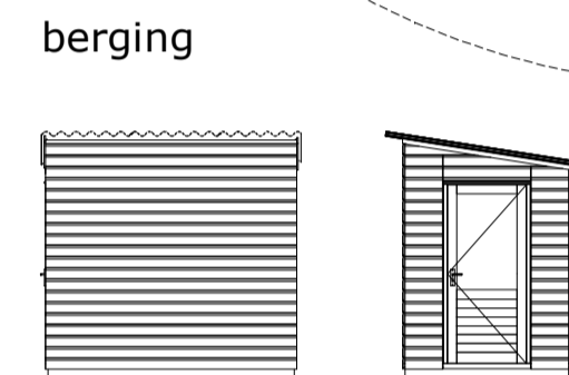
voor- en zijaanzicht 1 : 100
