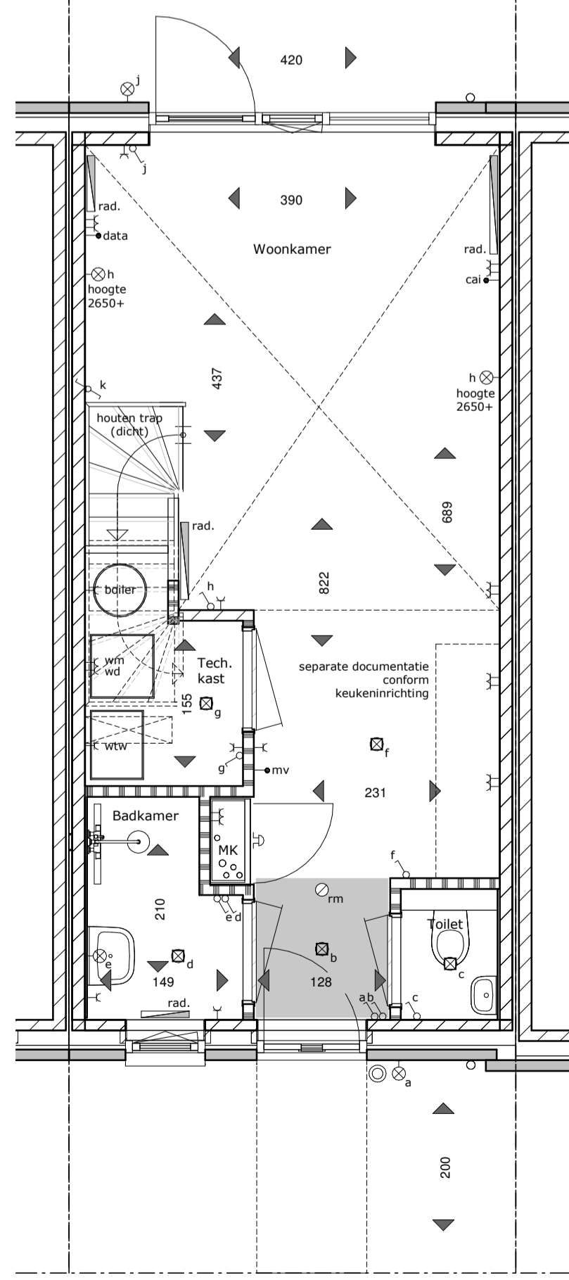
begane grond 1 : 50
