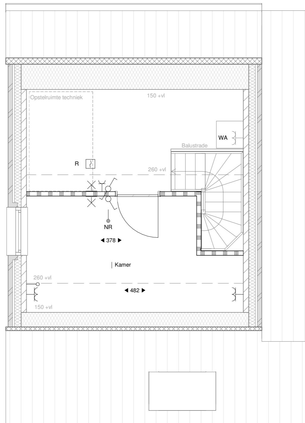
Tweede verdieping 1:50
