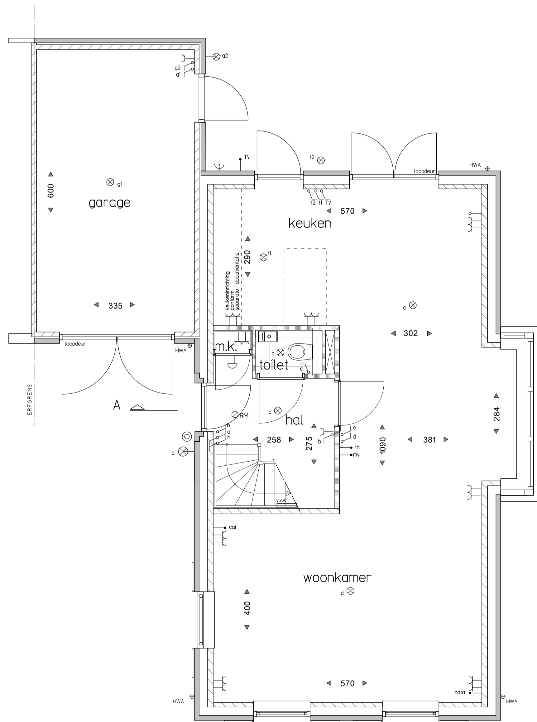
Begane grond
