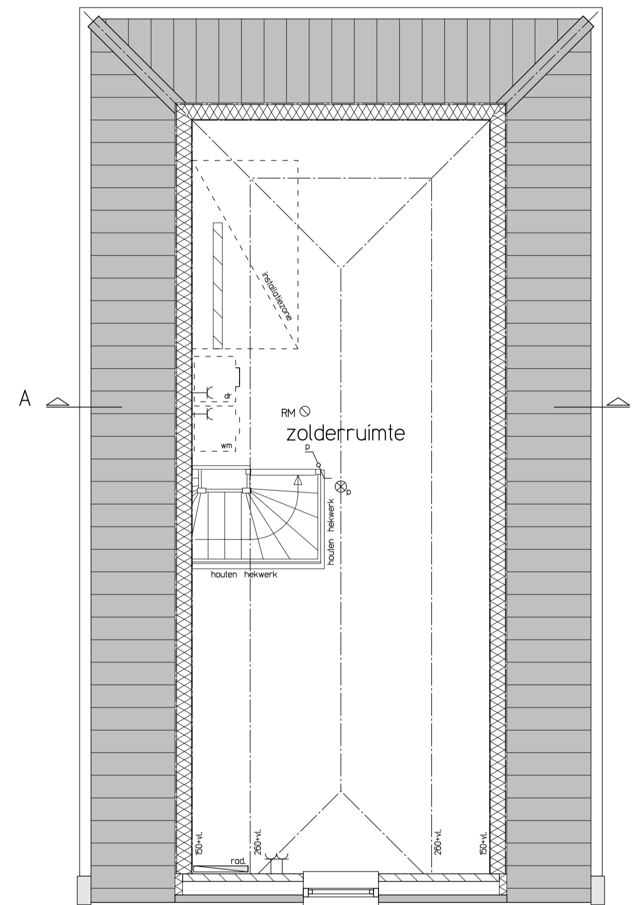
Tweede verdieping
