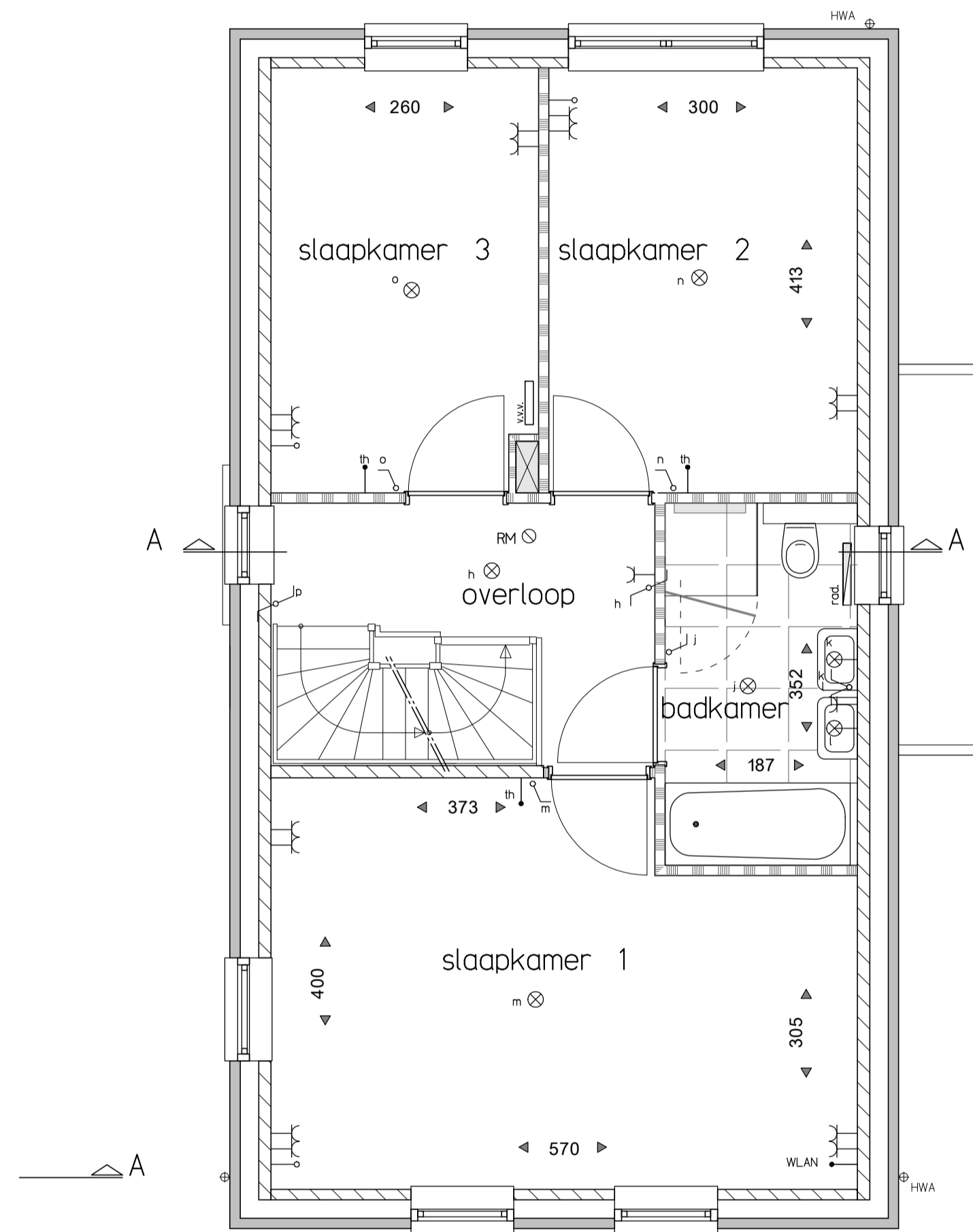
Eerste verdieping
