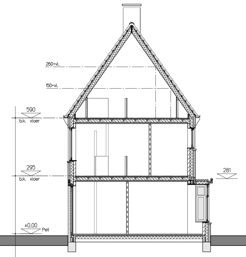
Doorsnede A-A
