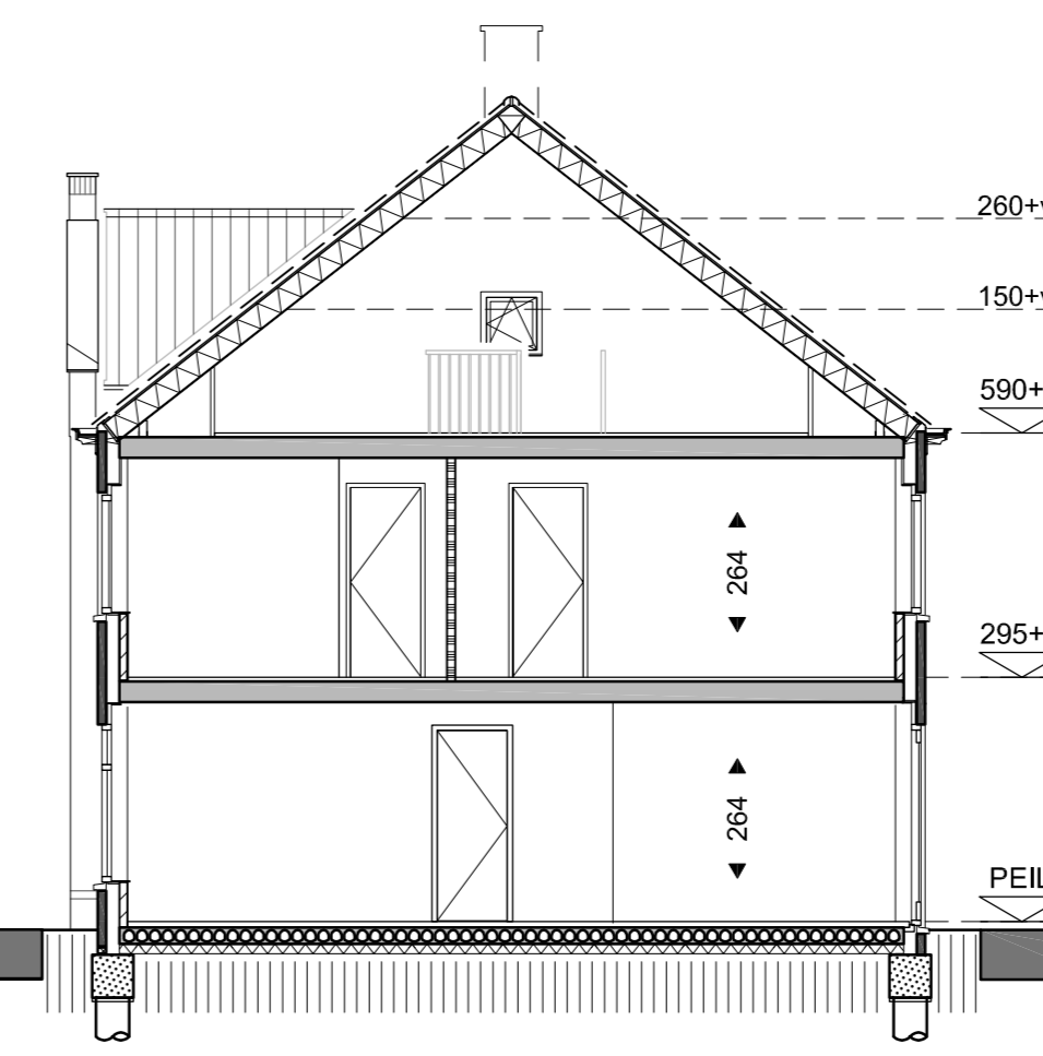
Doorsnede
