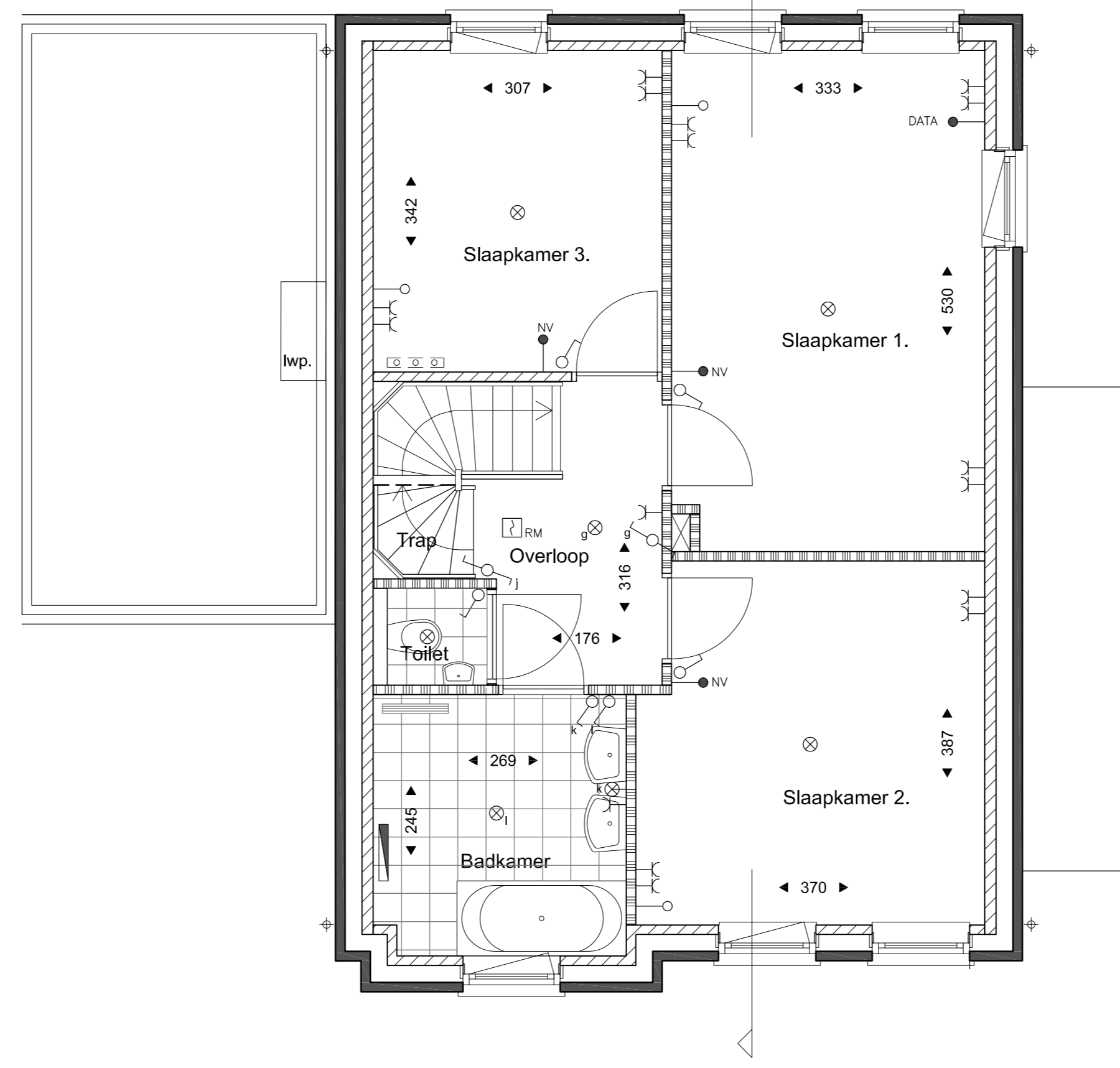
1e Verdieping Type A
