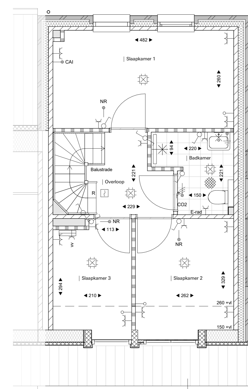
Eerste verdieping 1:100
