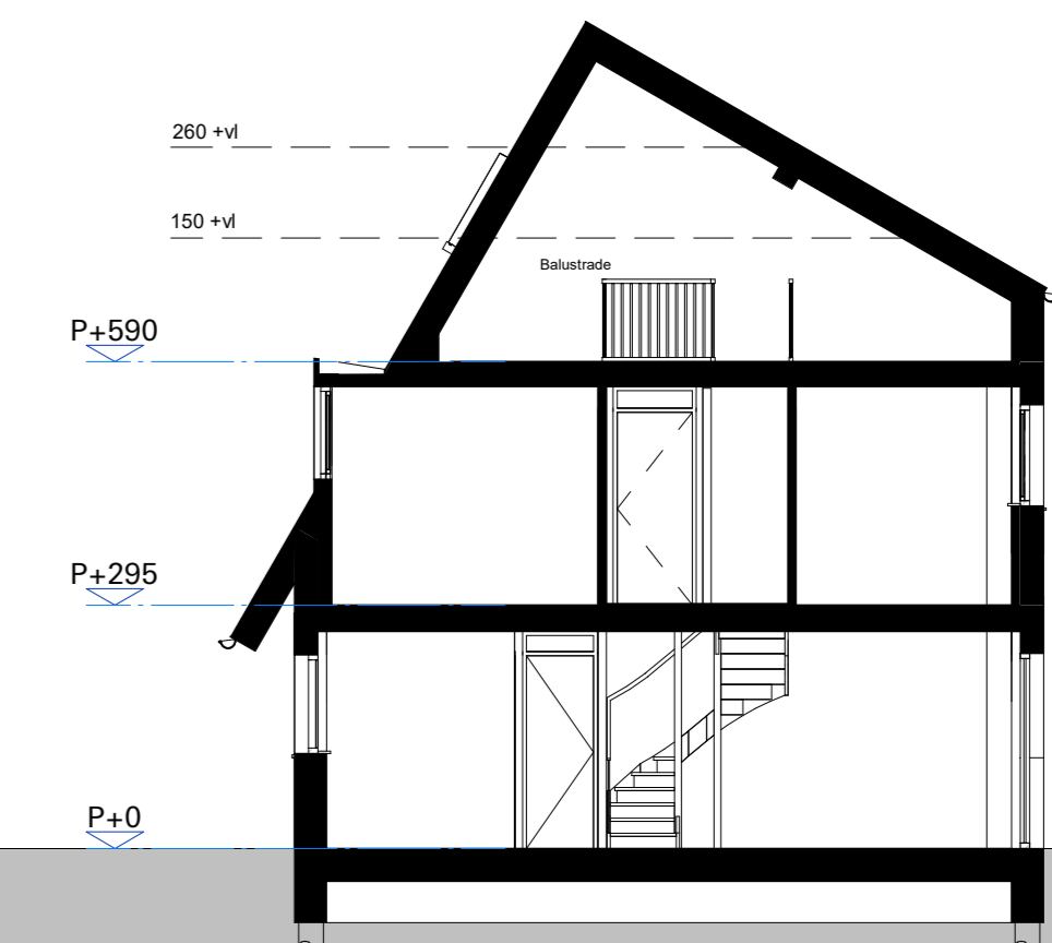
Doorsnede AA 1:100
