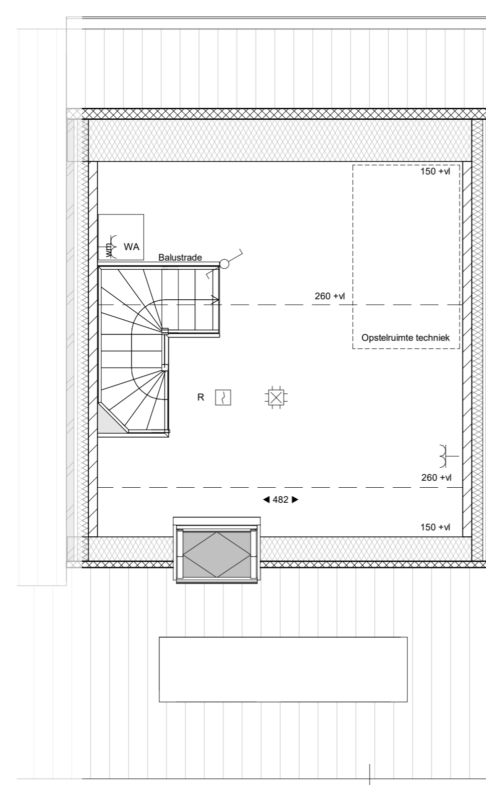
Tweede verdieping 1:100
