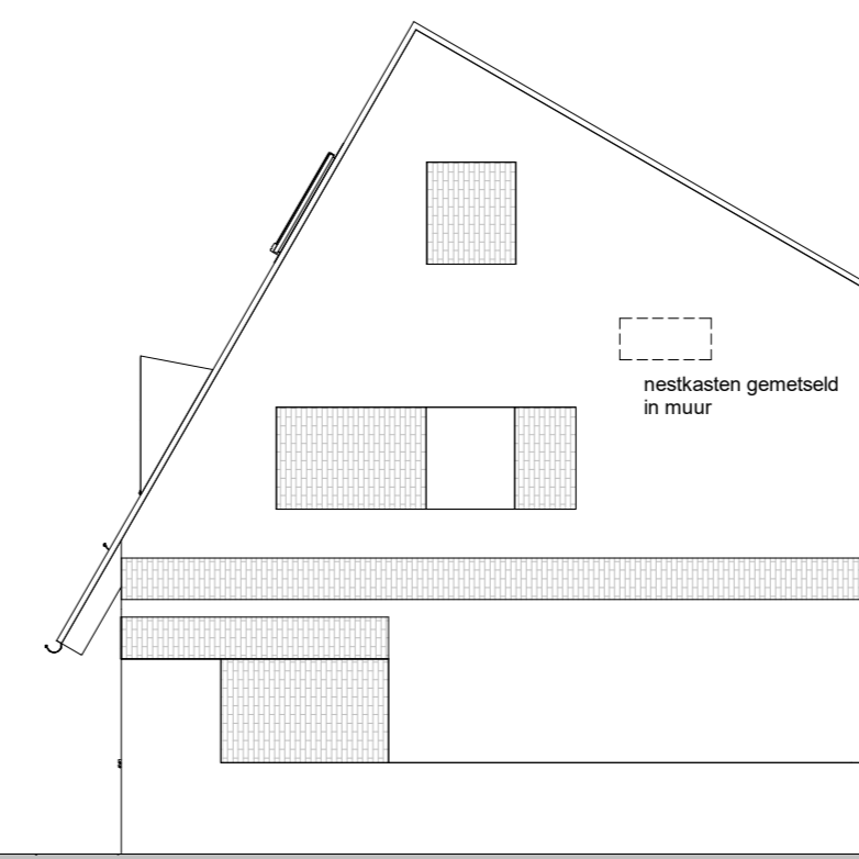
Rechterzijgevel 1:100
