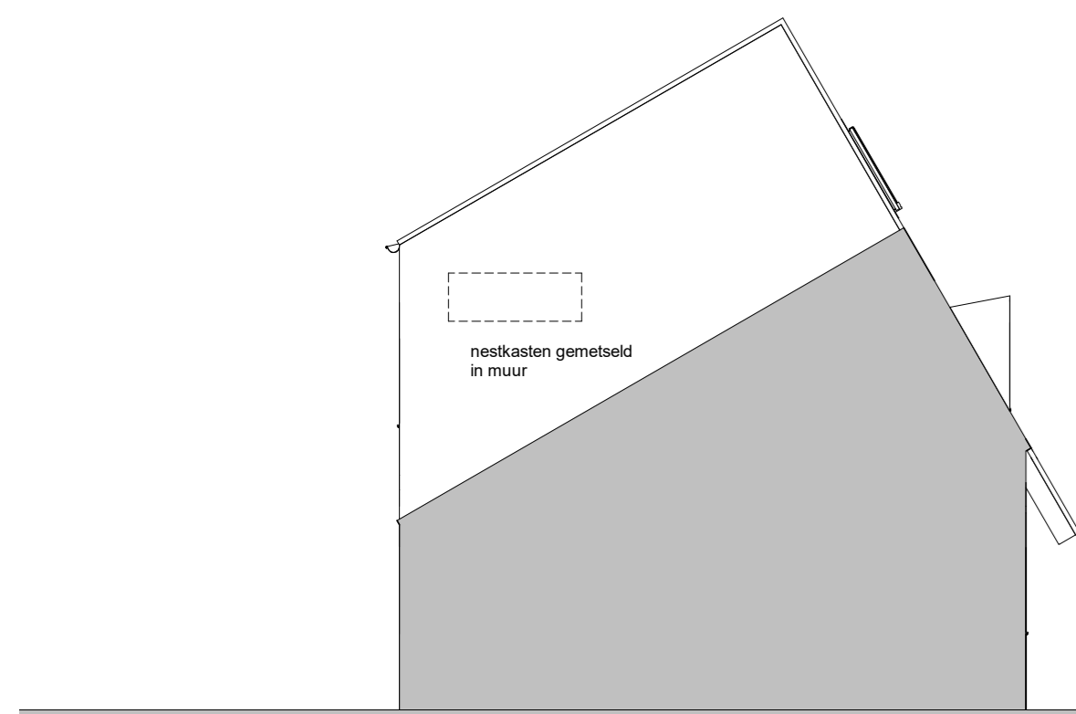
Linkerzijgevel 1:100
