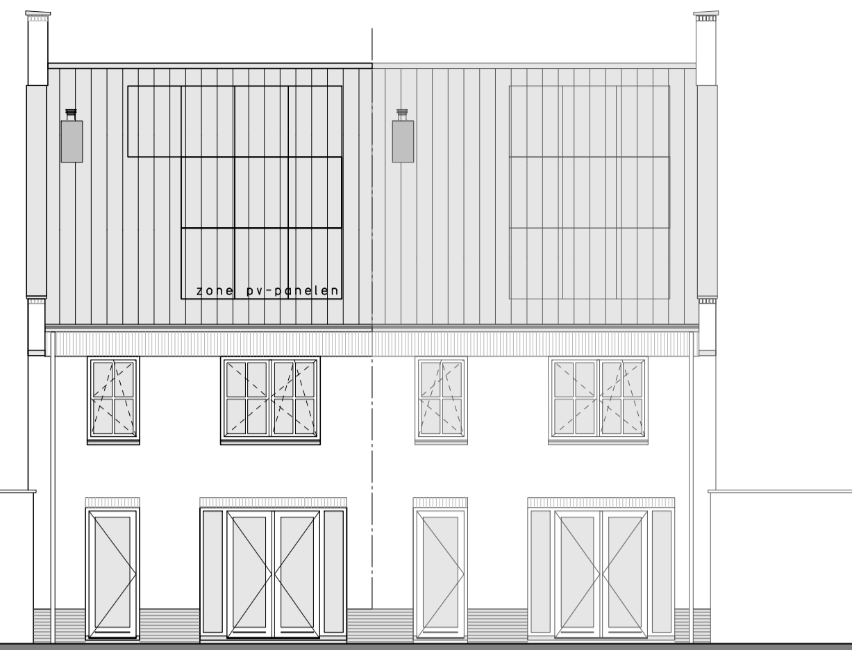
Achtergevel
