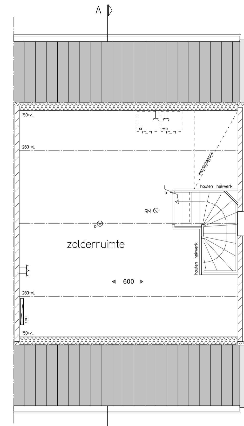
Tweede verdieping
