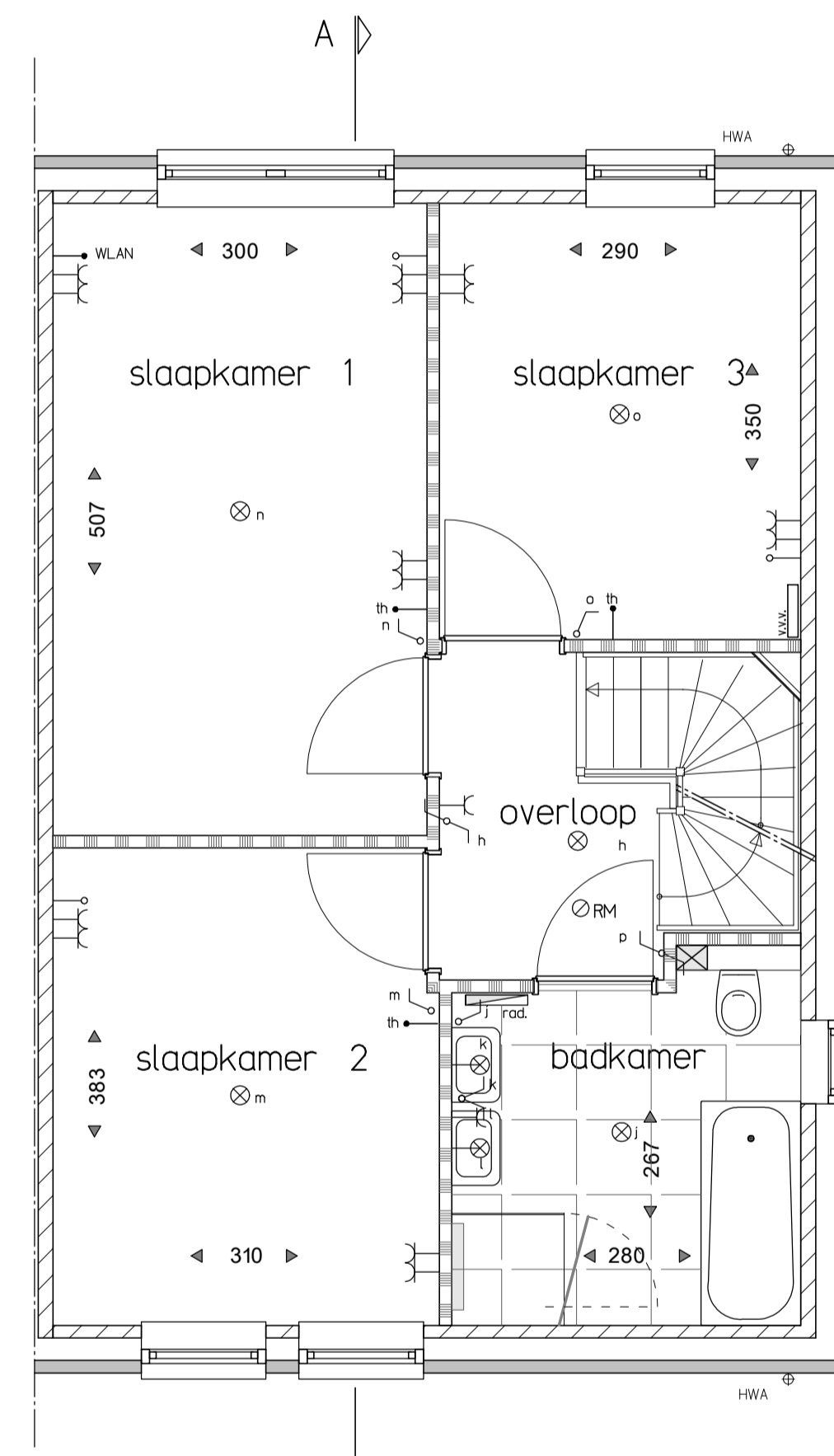
Eerste verdieping
