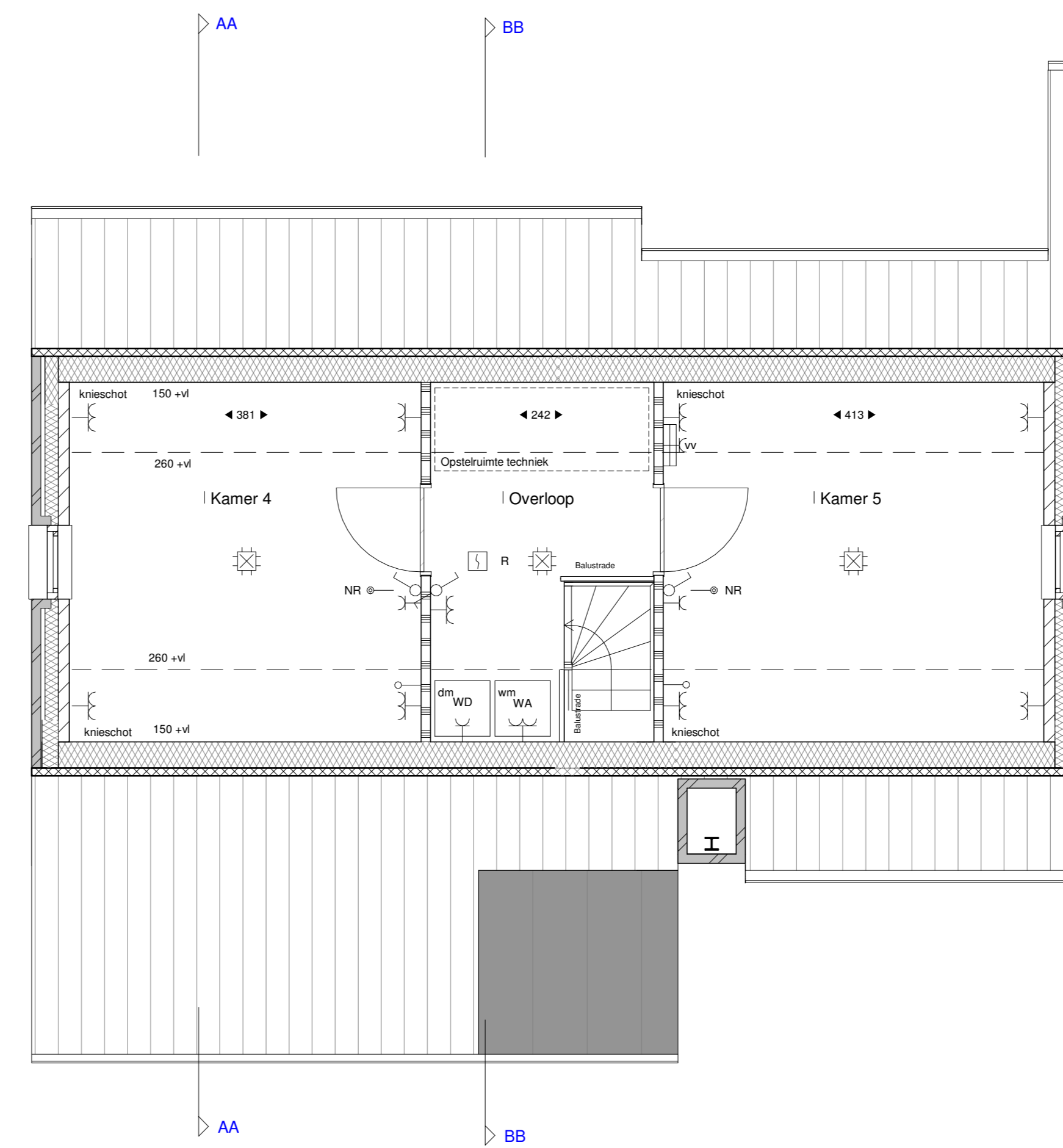
Eerste verdieping 1:100
