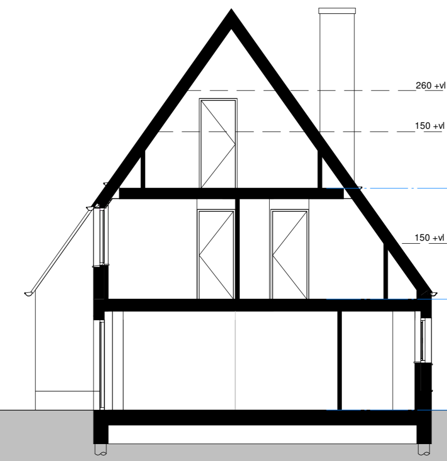
Doorsnede AA 1:100
