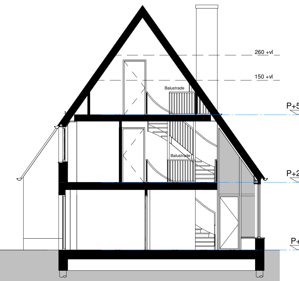
Doorsnede BB 1:100
