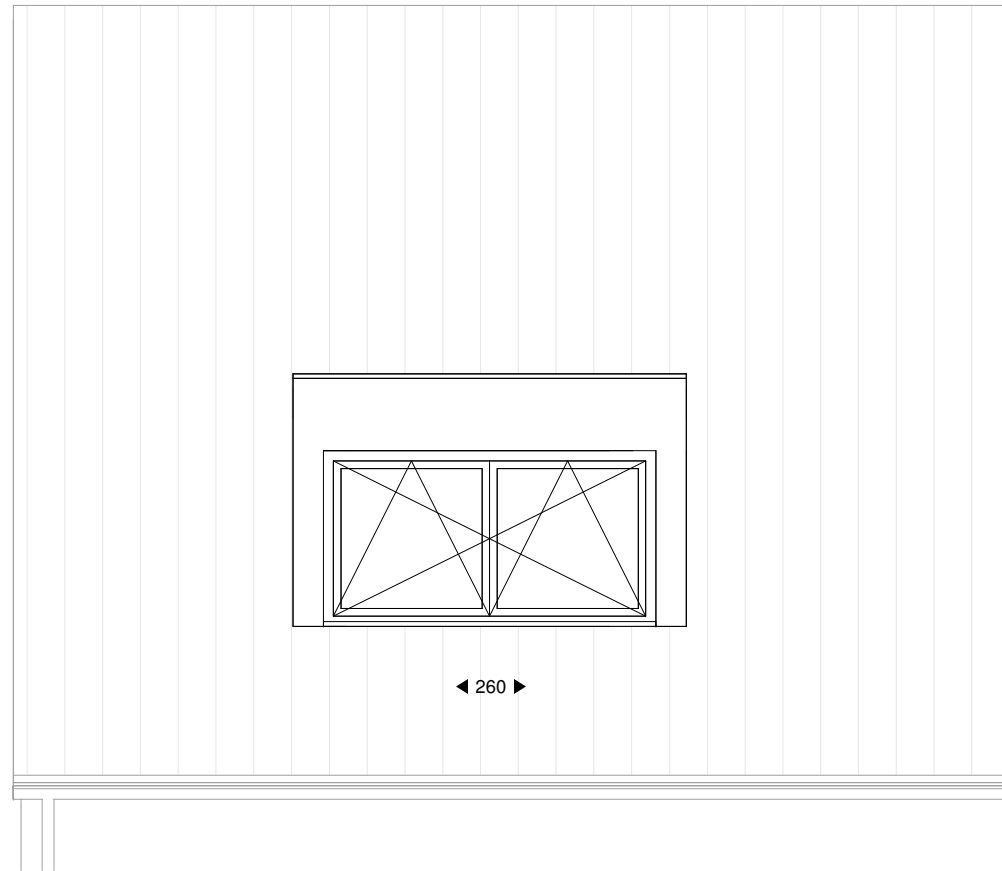
Dakkapel 220 cm inwendig. 1:50
