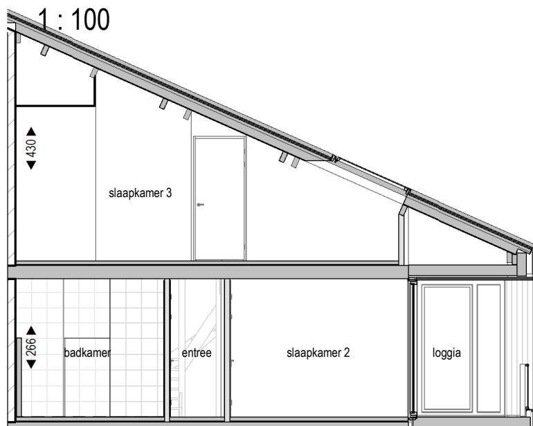
doorsnede
