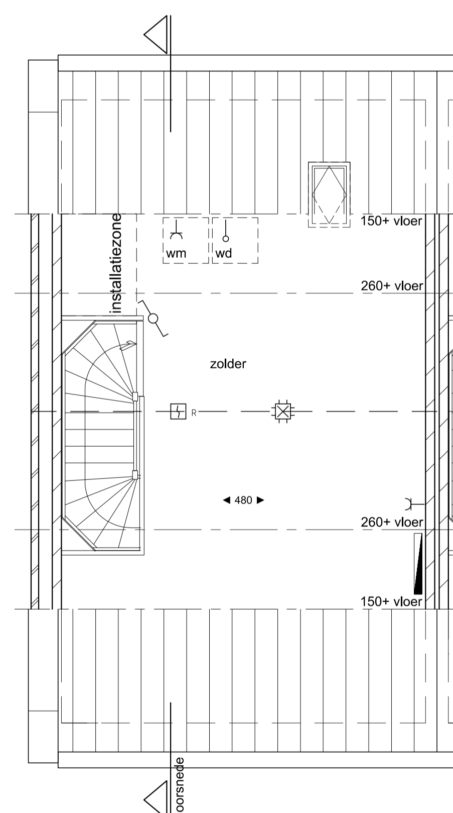
2e Verdieping type O BNR 132
