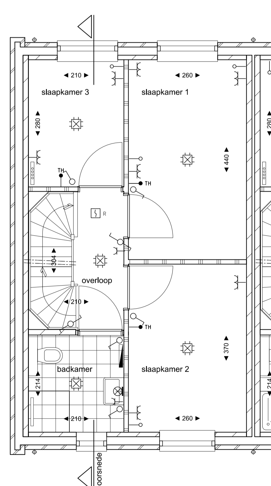
1e Verdieping type O BNR 132
