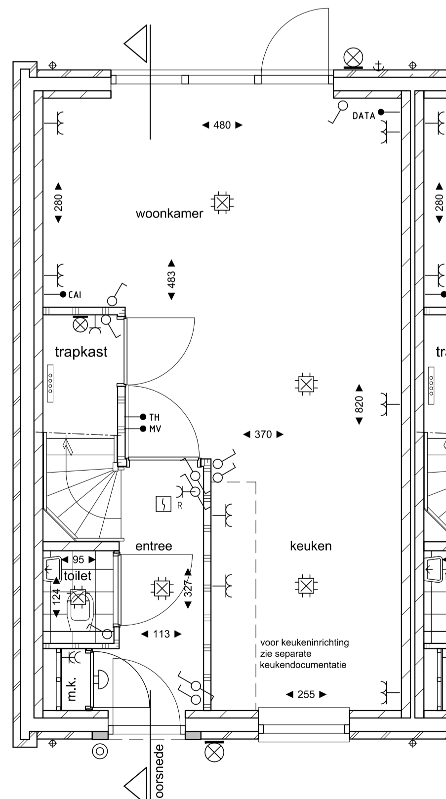
Begane grond type O BNR 132
