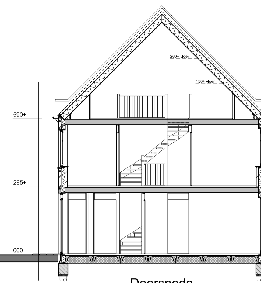
Doorsnede
