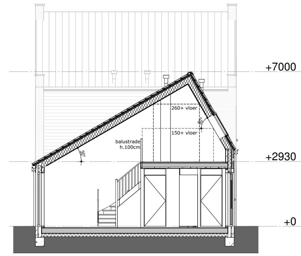
doorsnede 1 : 100
