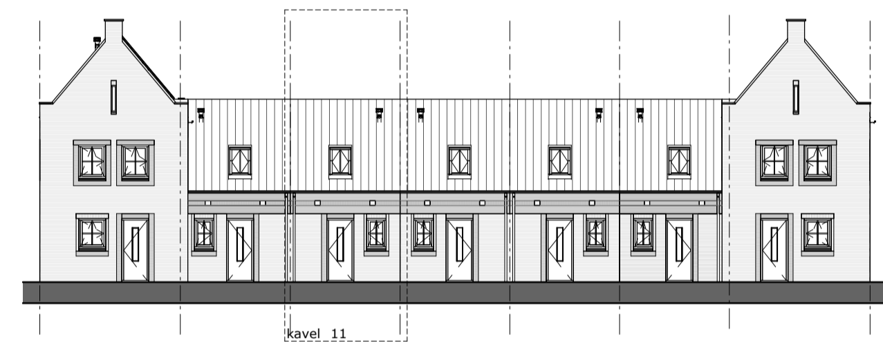
voorgevel
