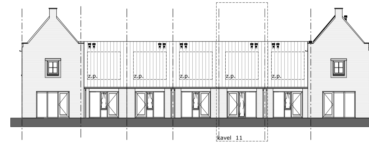
achtergevel
