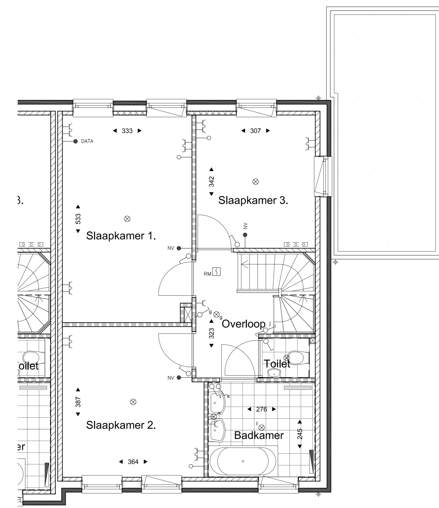
1e Verdieping Type G kavel 21
