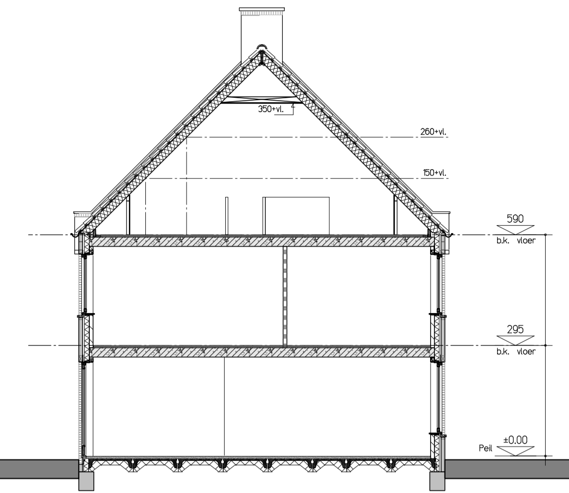
Doorsnede A-A
