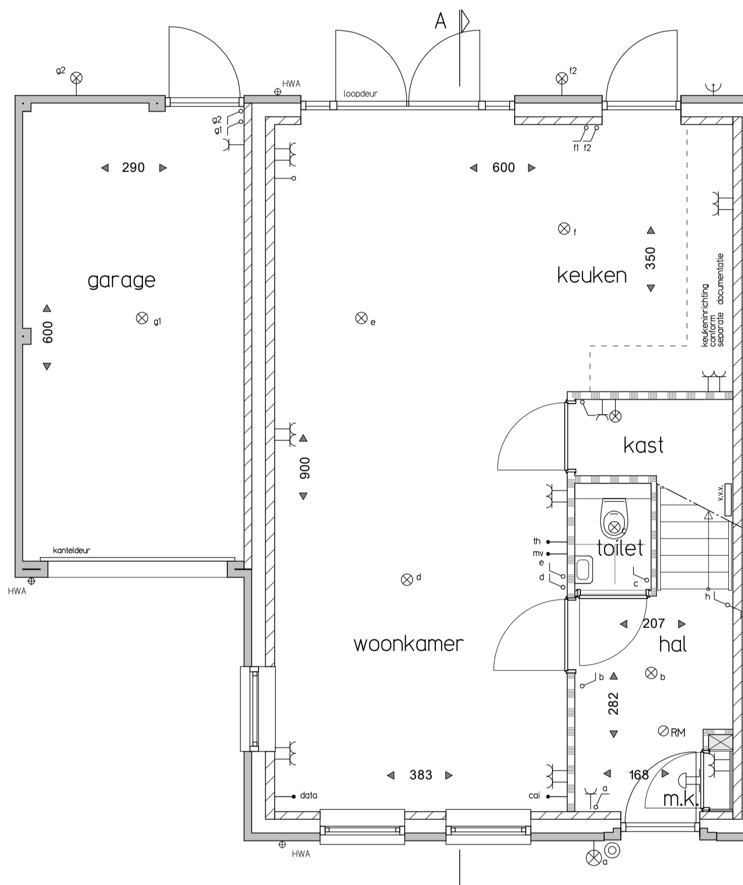
Begane grond
