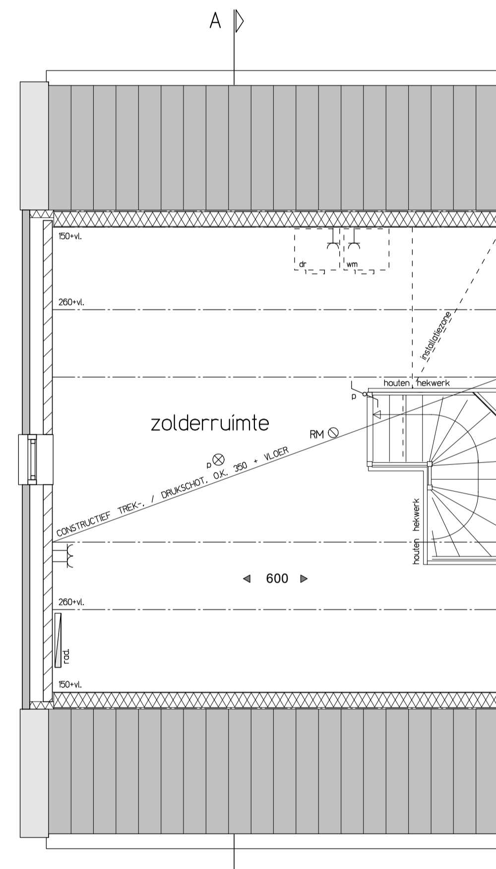
Tweede verdieping
