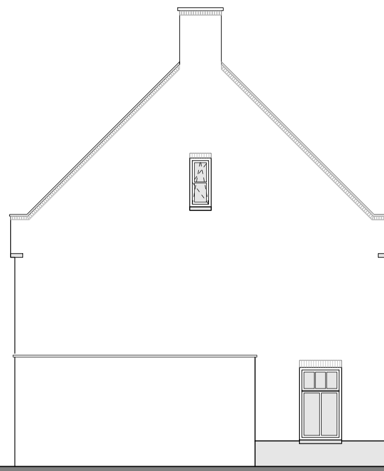
Linker zijgevel
