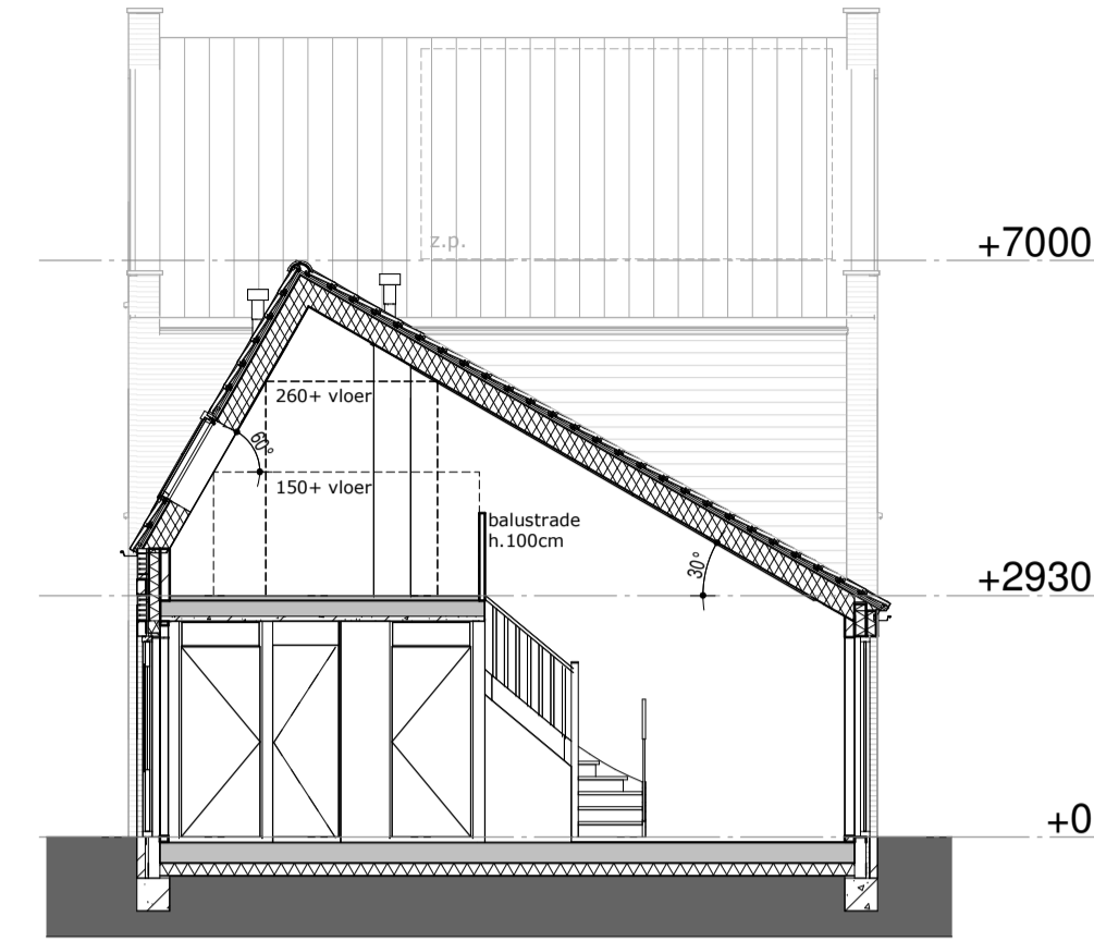
doorsnede 1 : 100
