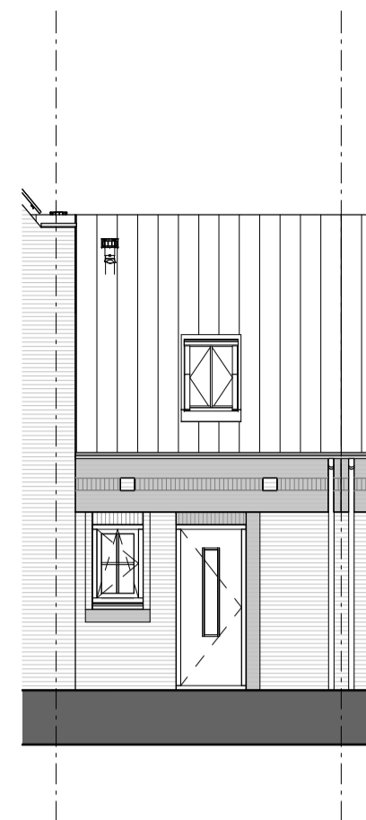
voorgevel 1 : 100
