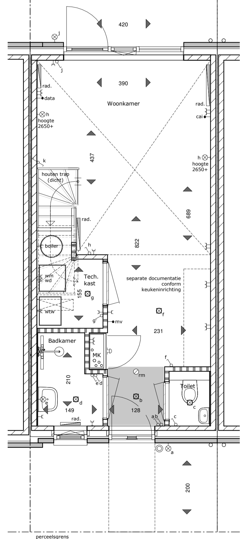
begane grond 1 : 50
