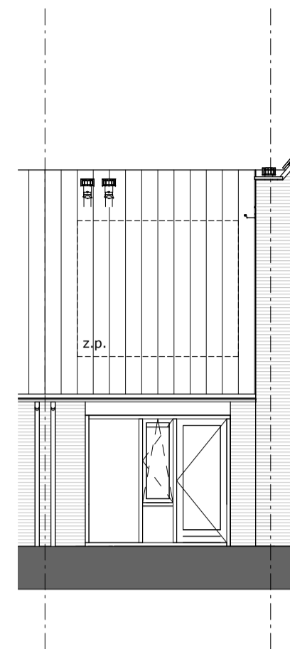
achtergevel 1 : 100
