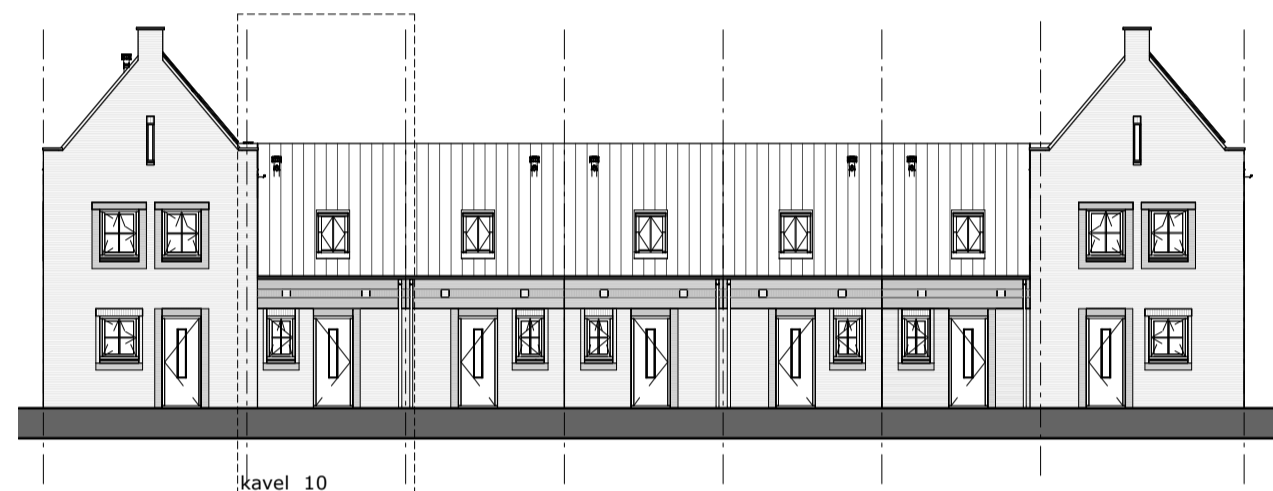
voorgevel
