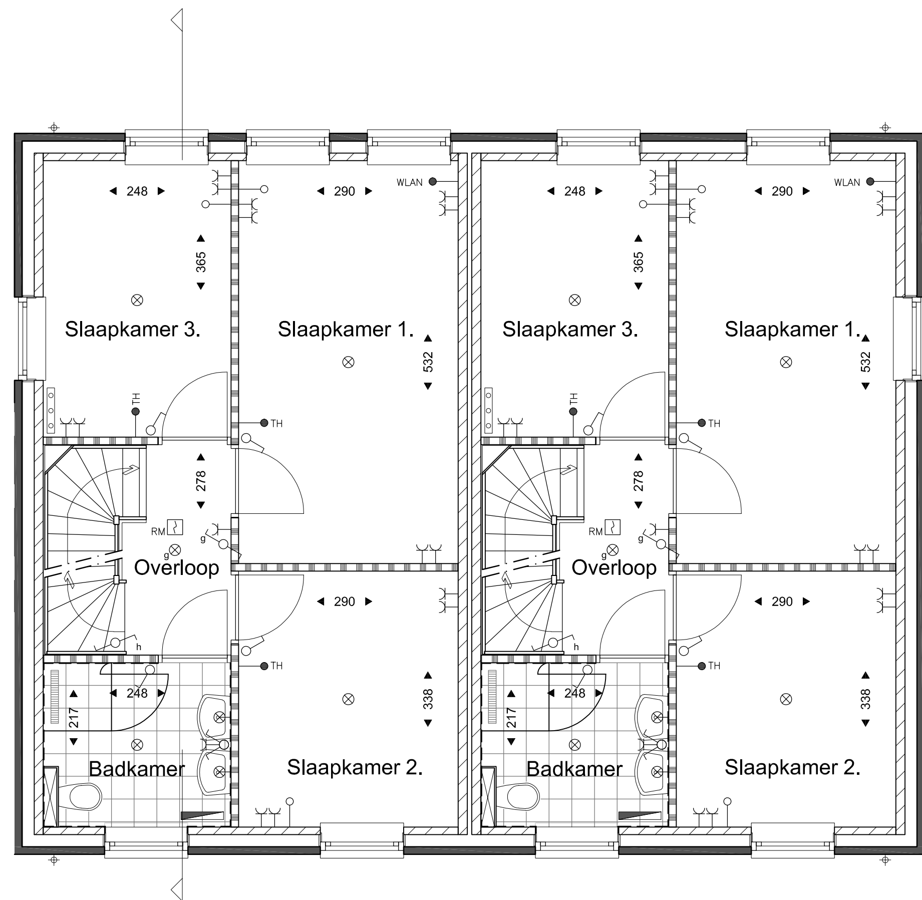
1e Verdieping
