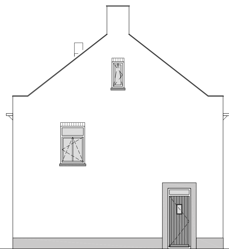
Linker zijgevel kavel 44
