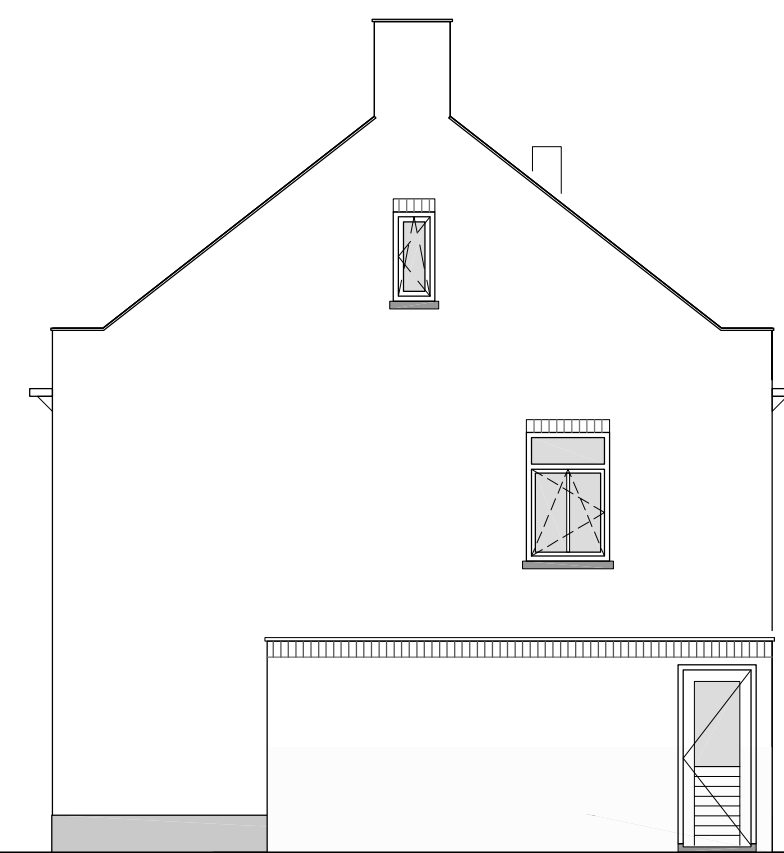
Rechter zijgevel kavel 45
