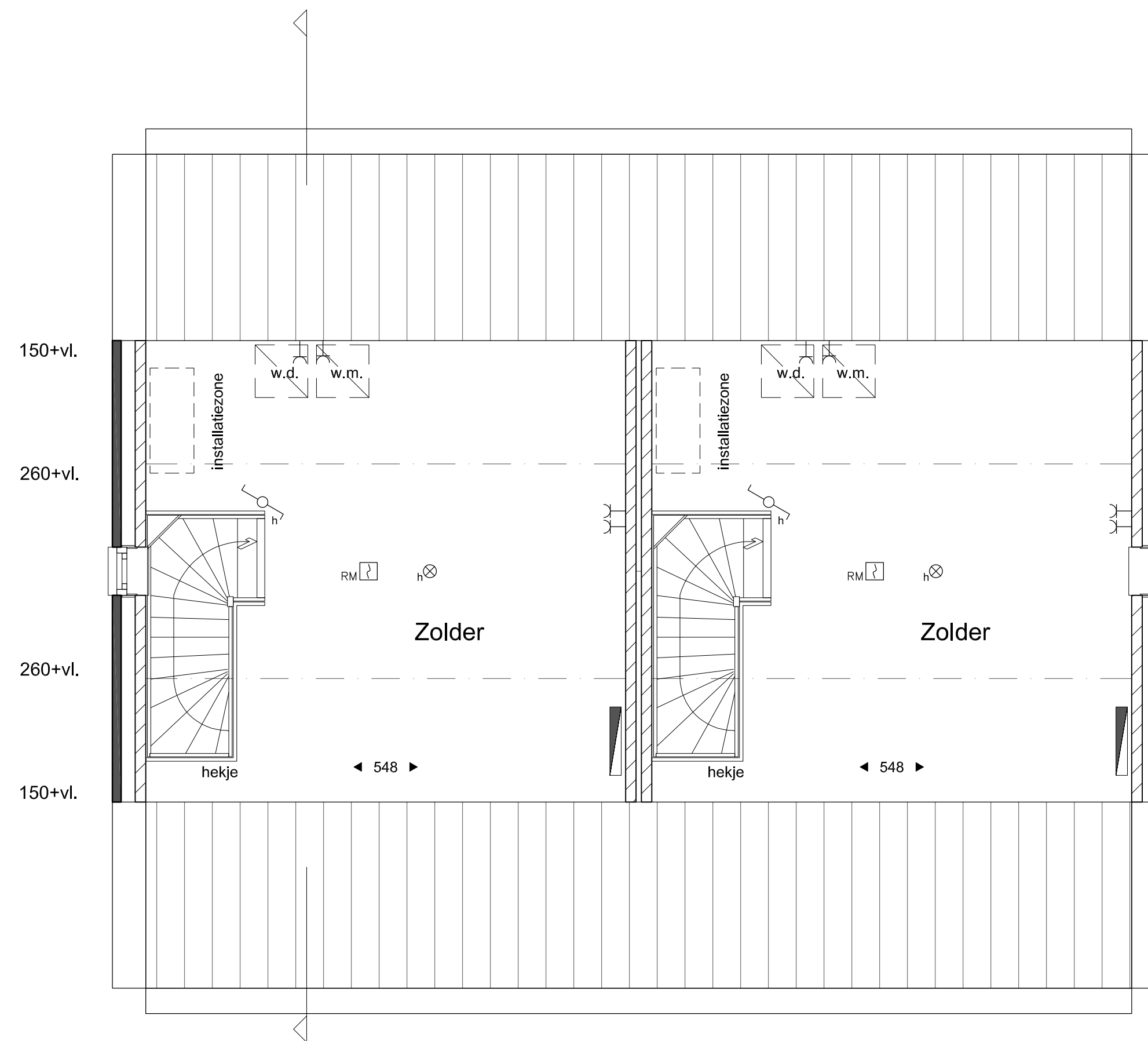
2e Verdieping
