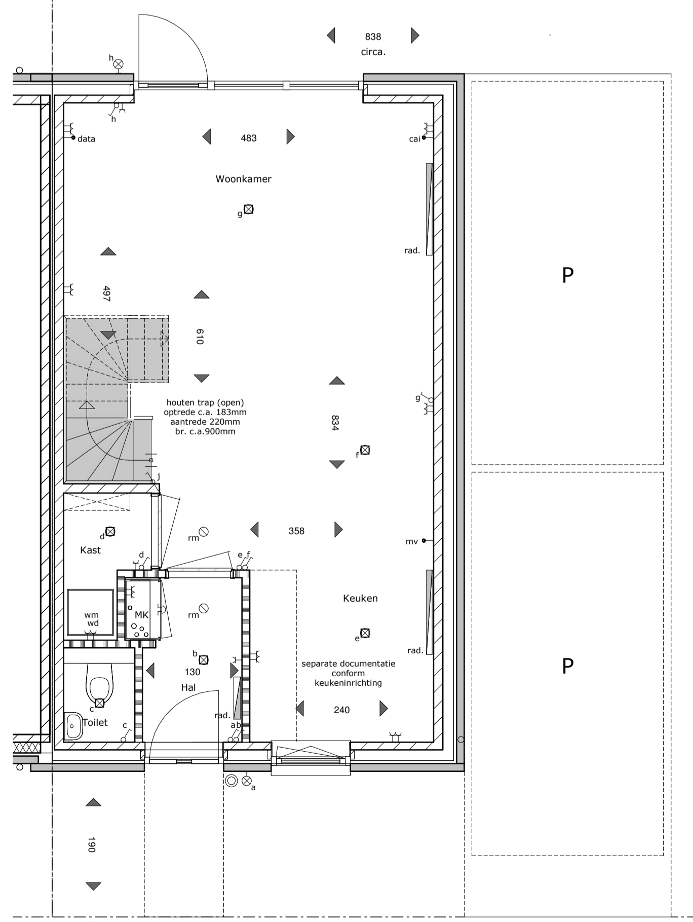
begane grond 1 : 50
