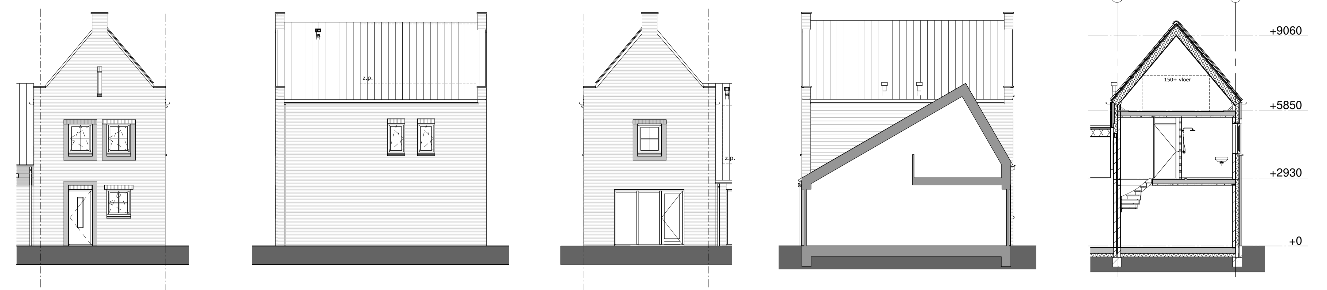
linkergevel 1 : 100
