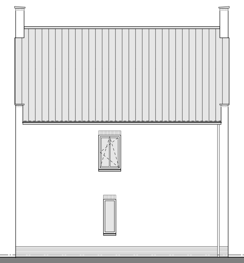
Linker zijgevel bouwnummer 111
