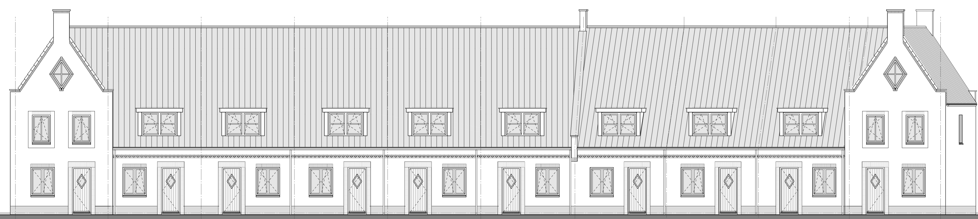
Voorgevel bouwnummer 97 t/m 106
