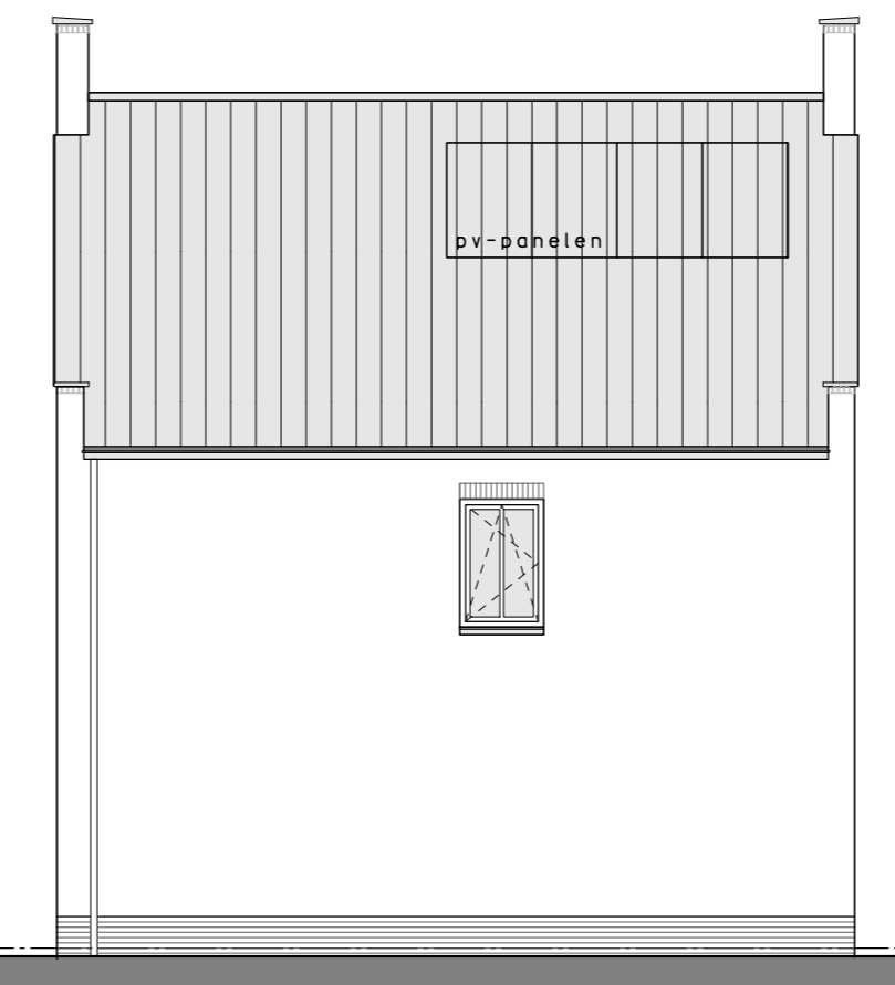
Rechter zijgevel bouwnummer 97 en 112
