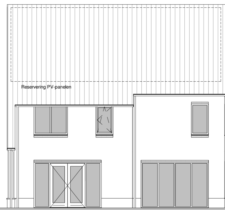
Achtergevel 1:100
