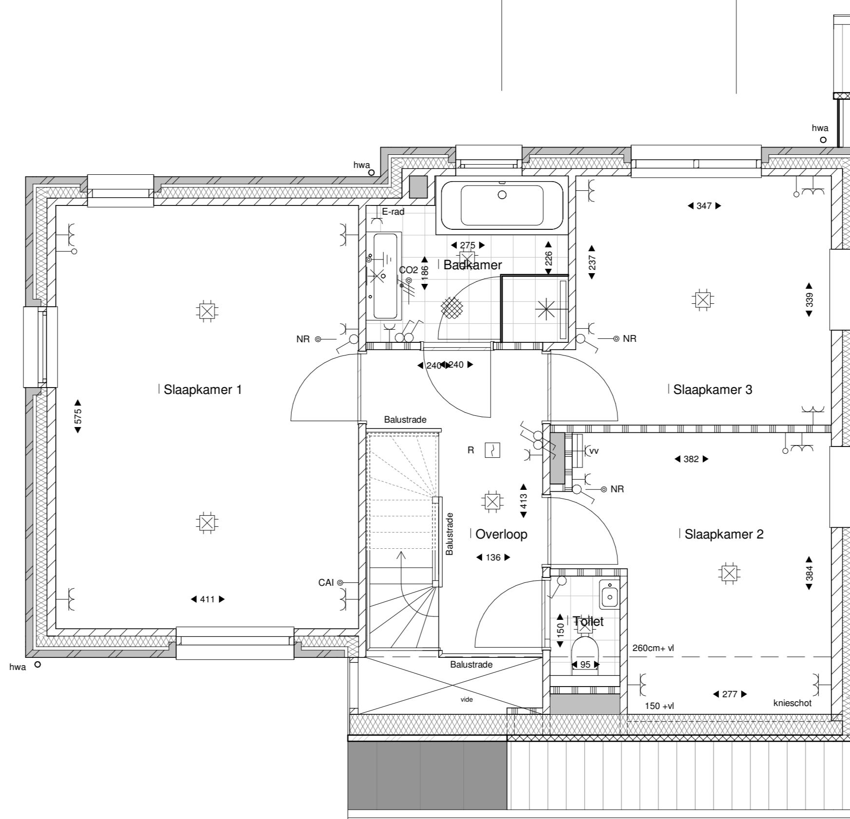
Tweede verdieping 1:50
