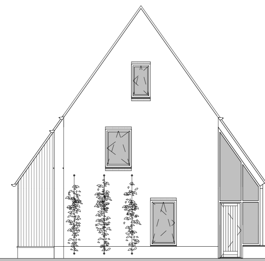
Linkerzijgevel 1:100
