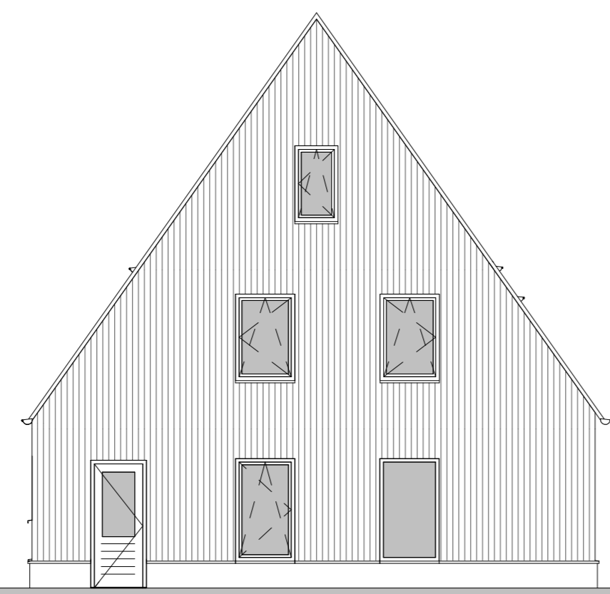
Rechterzijgevel 1:100
