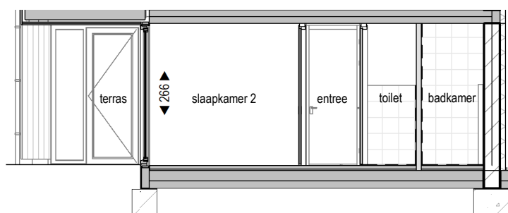
doorsnede
