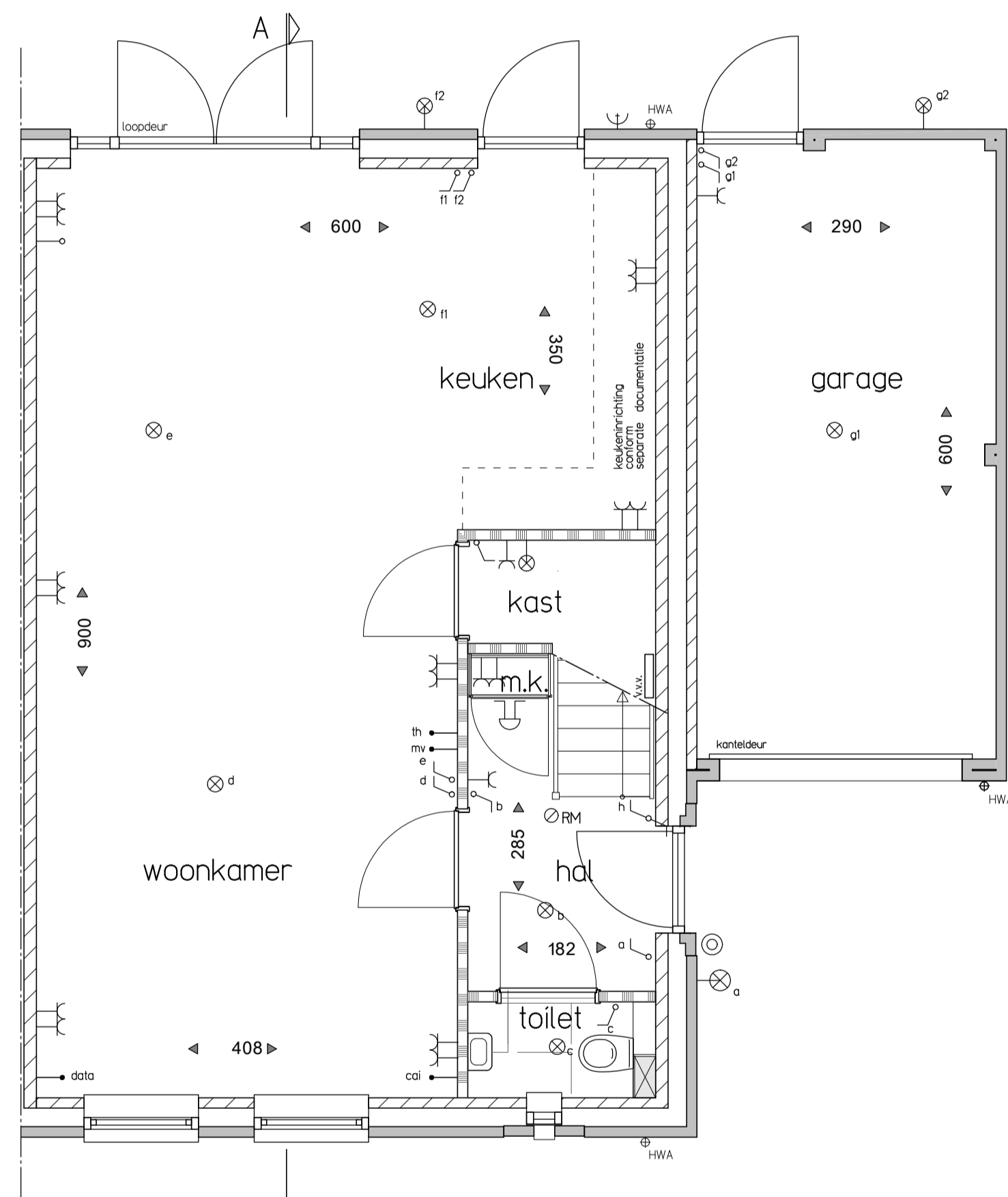
Begane grond
