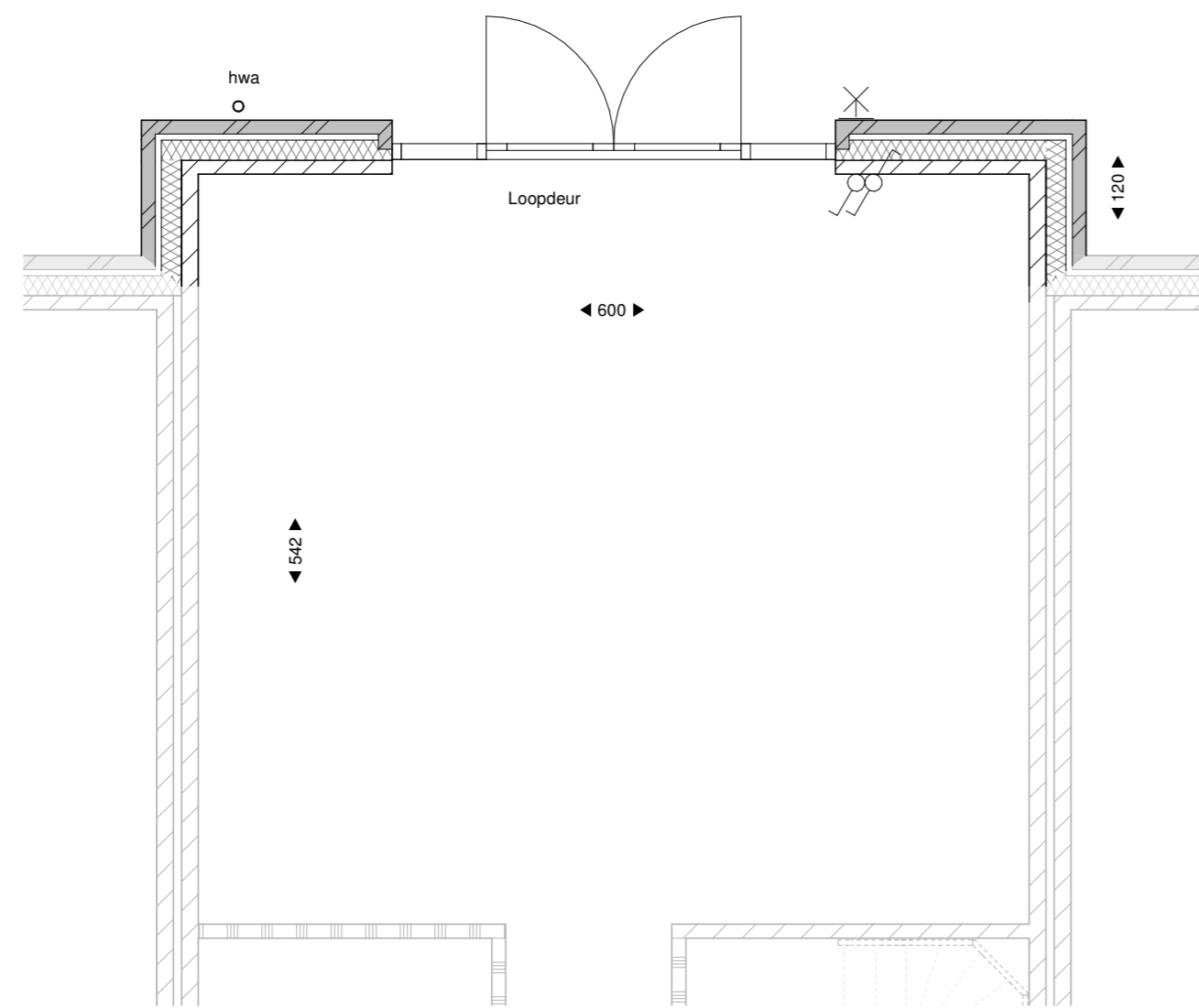
Begane grond 1:50
