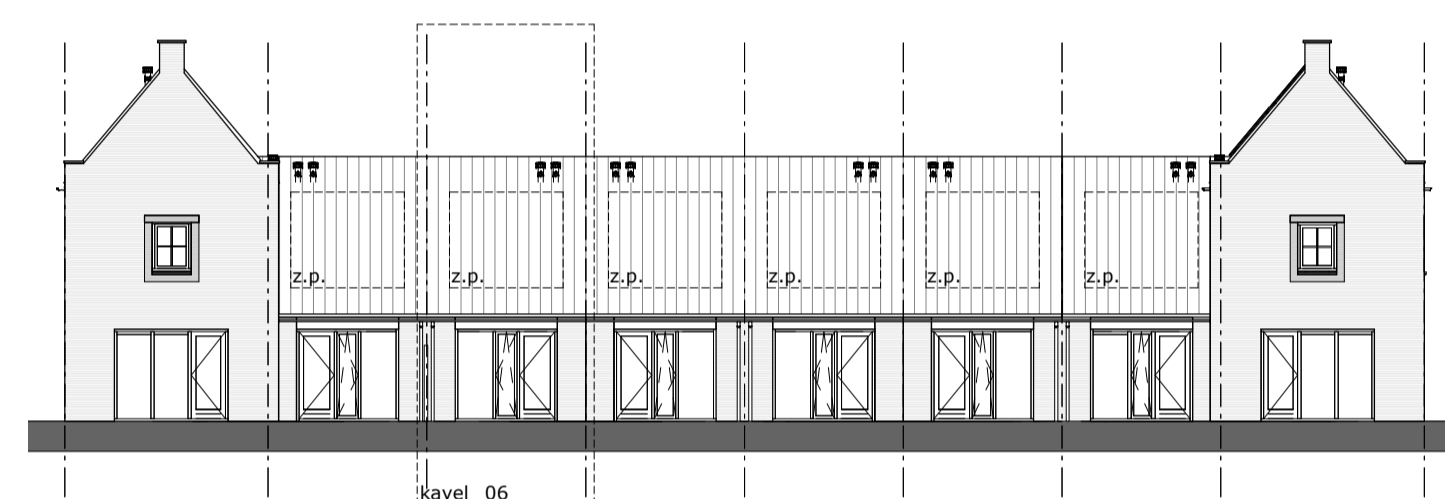
achtergevel
