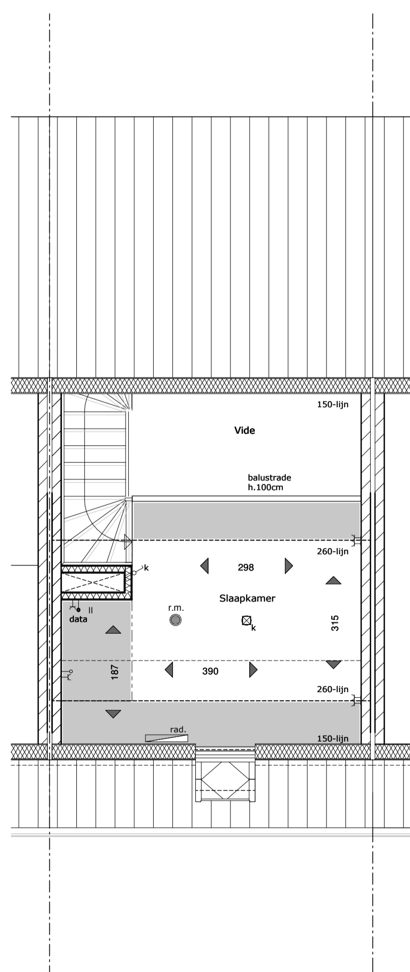
eerste verdieping 1 : 50
