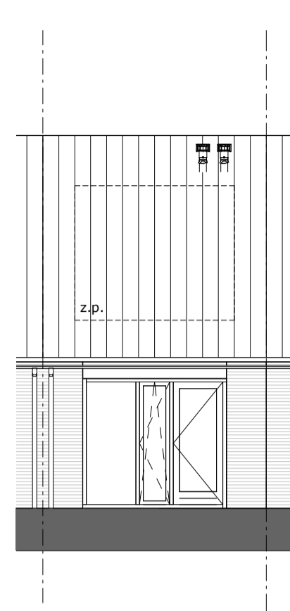
achtergevel 1 : 100
