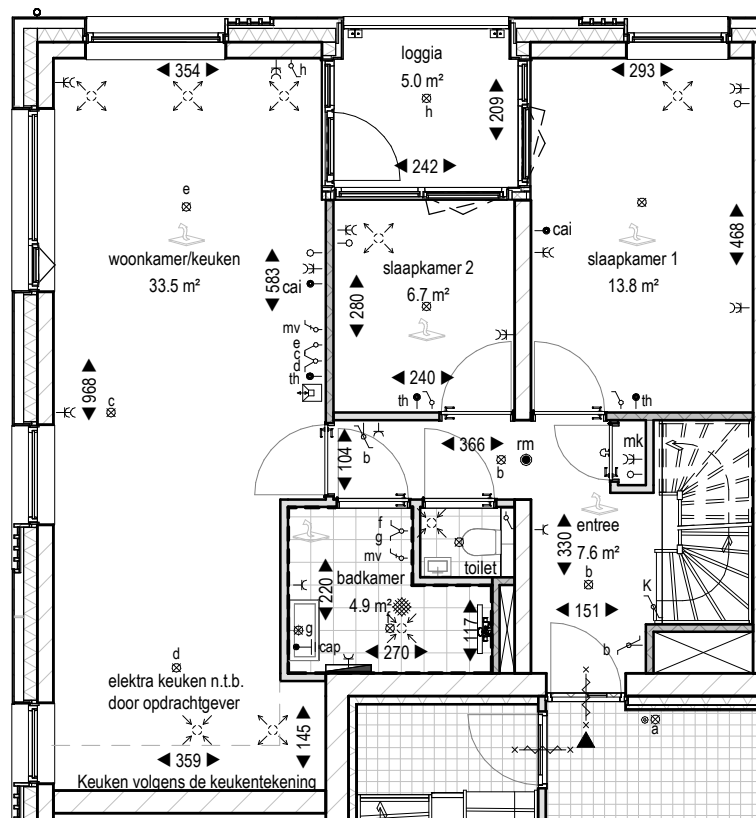
plaattegrond woonlaag 1
